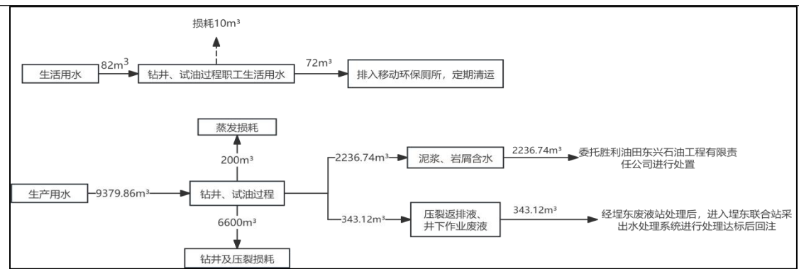
图 2-2 项目水平衡图
