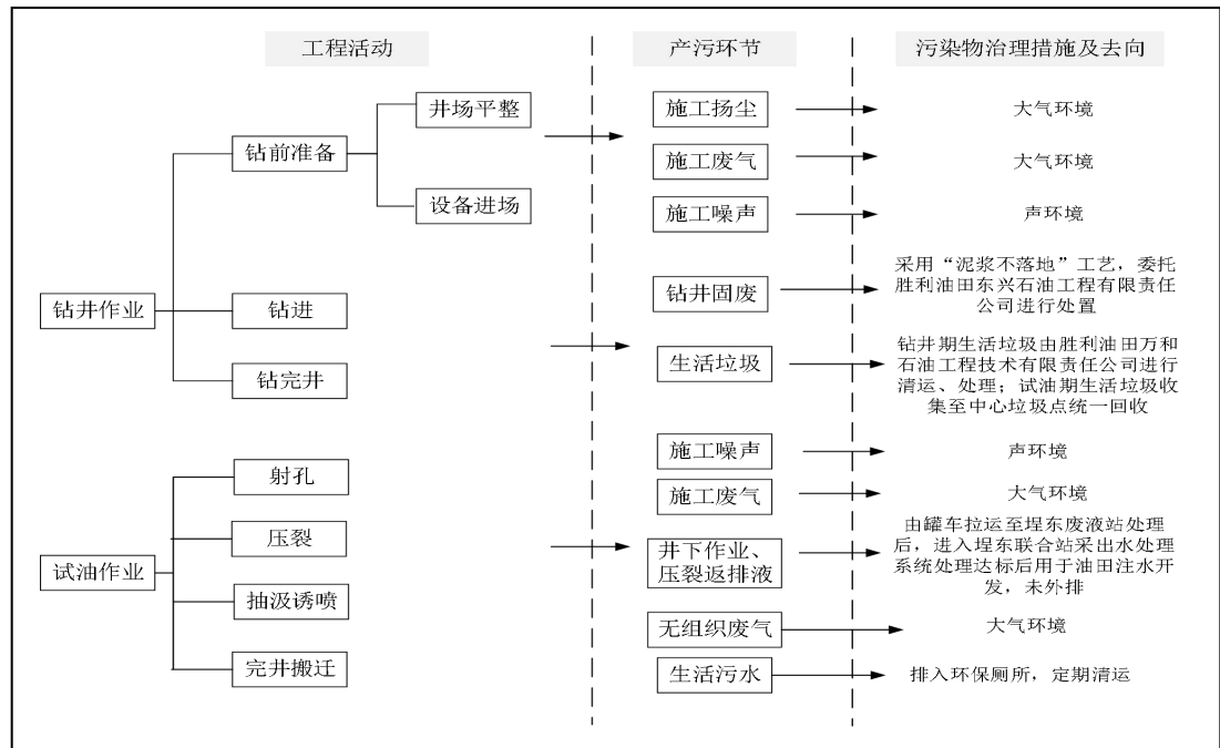
图 2-8 钻井及试油工艺流程及产污环节图
