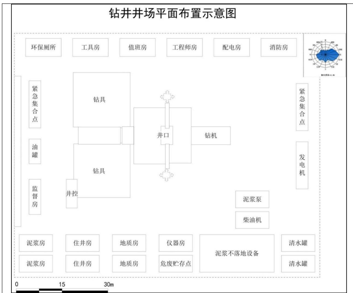
图 2-6 钻井井场平面布置示意图
