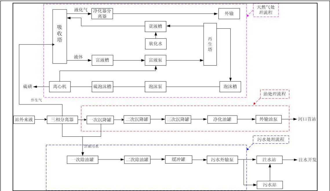
图 2-4 埕东联合站工艺流程图
