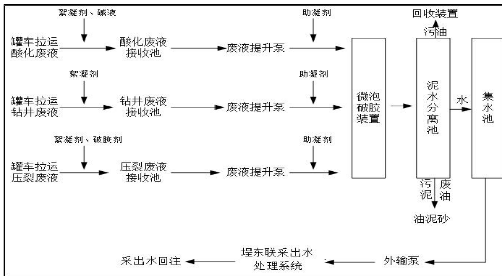
图 2-3 埕东废液处理站工艺流程图
