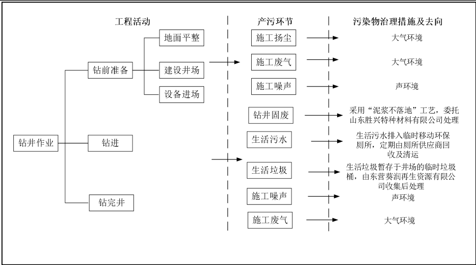
图 2-6 钻井工艺流程及产污环节图
