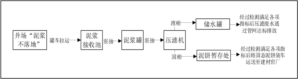
图 2-3 山东胜兴特种材料有限公司泥浆处置工艺流程示意图
