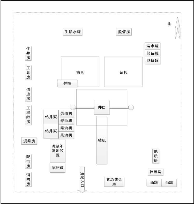
图 2-5 钻井井场平面布置示意图
