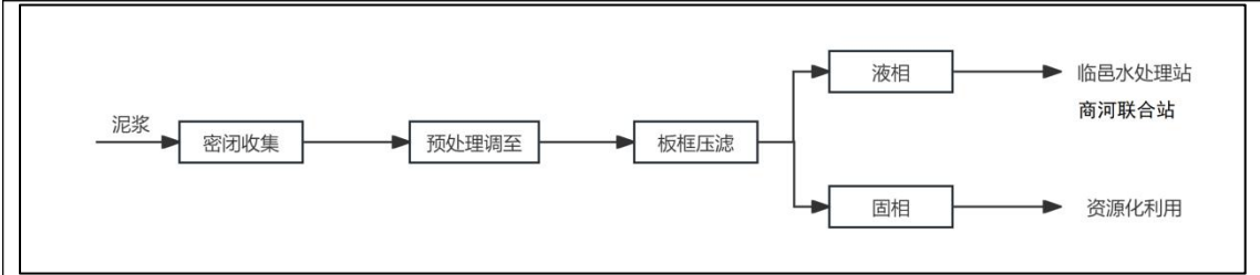
图 2-1 胜利油田德利实业有限责任公司泥浆处理工艺流程图
