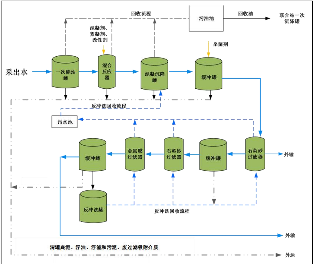
图 2-2 临二联合站采出水处理系统工艺流程图
