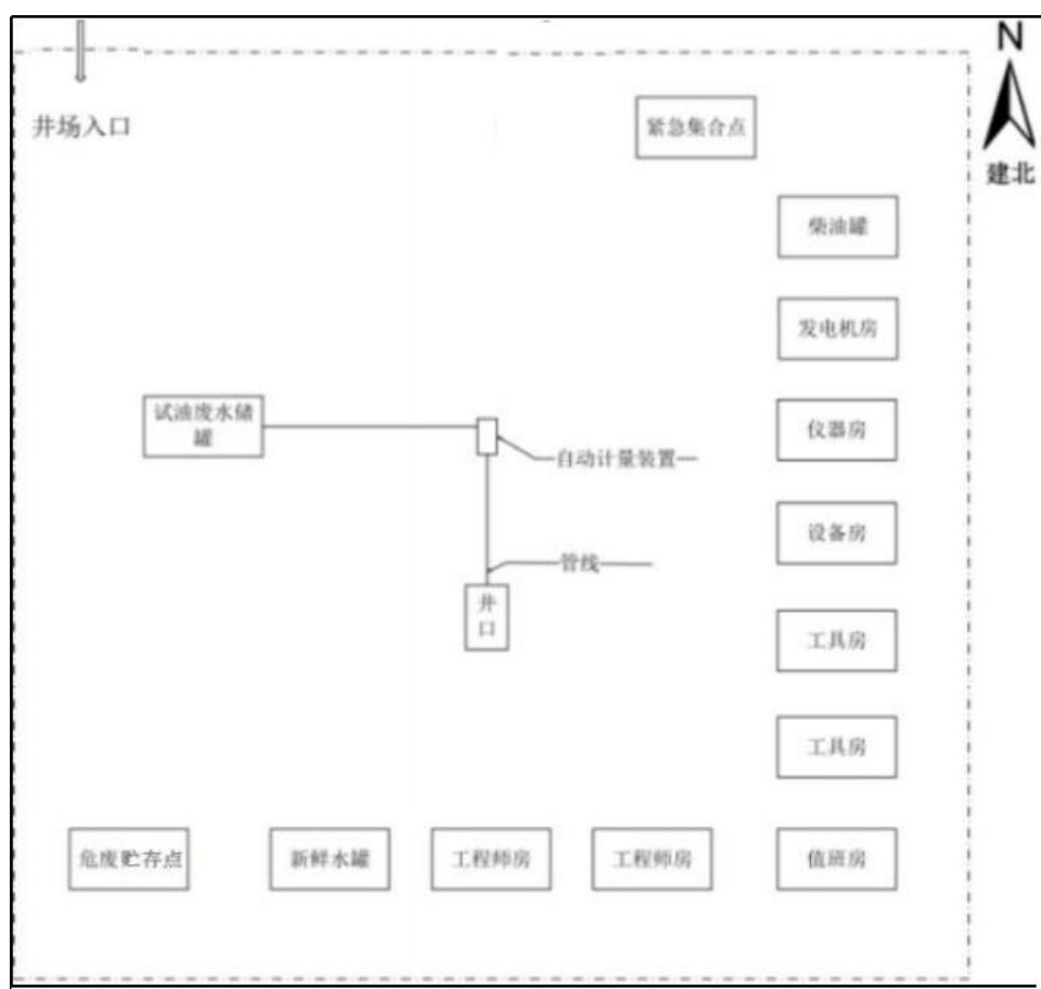
图 2-5 试油过程平面布置示意图
