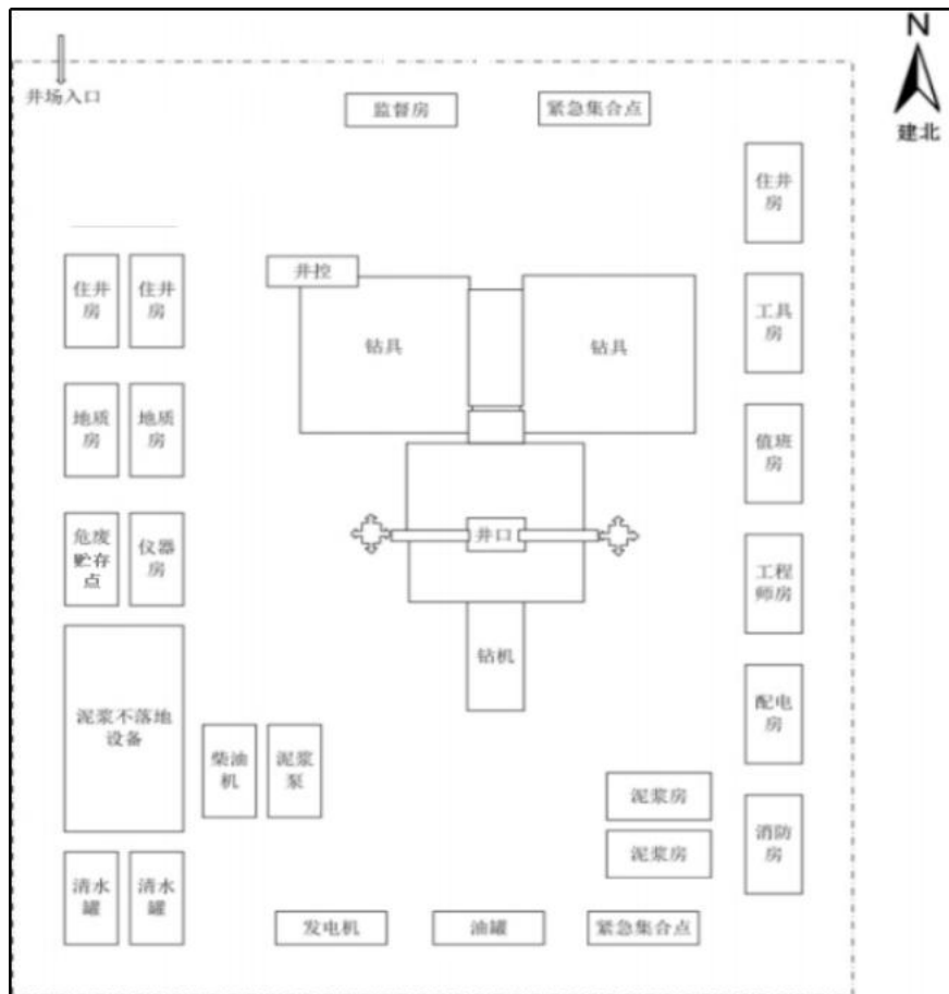
图 2-4 钻井井场平面布置示意图
