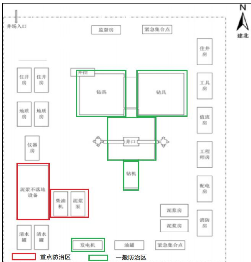
图 4-2 项目分区防渗图
