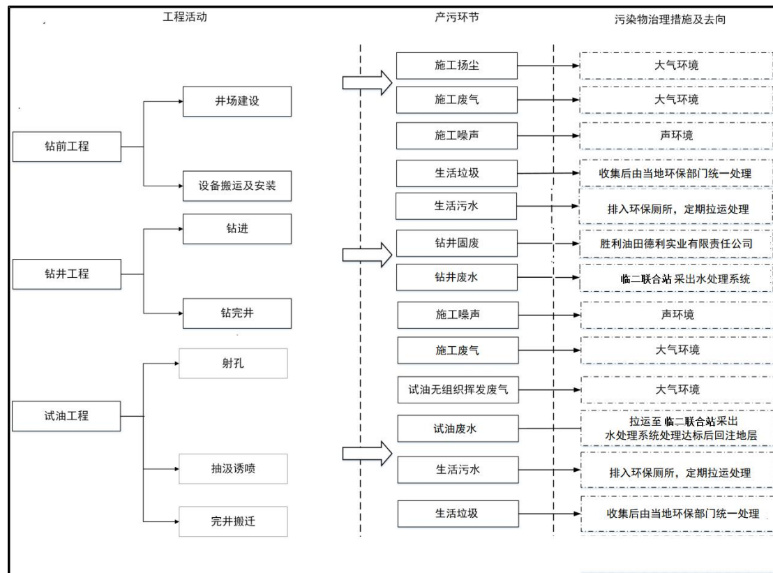
图 2-6 钻井及试油工艺流程及产污环节图
