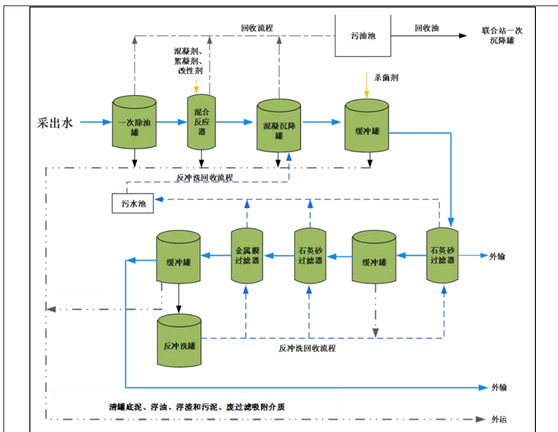
图 2-4 临二联合站采出水处理系统工艺流程图
