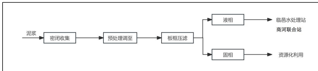
图 2-2 胜利油田德利实业有限责任公司泥浆处理工艺流程图
