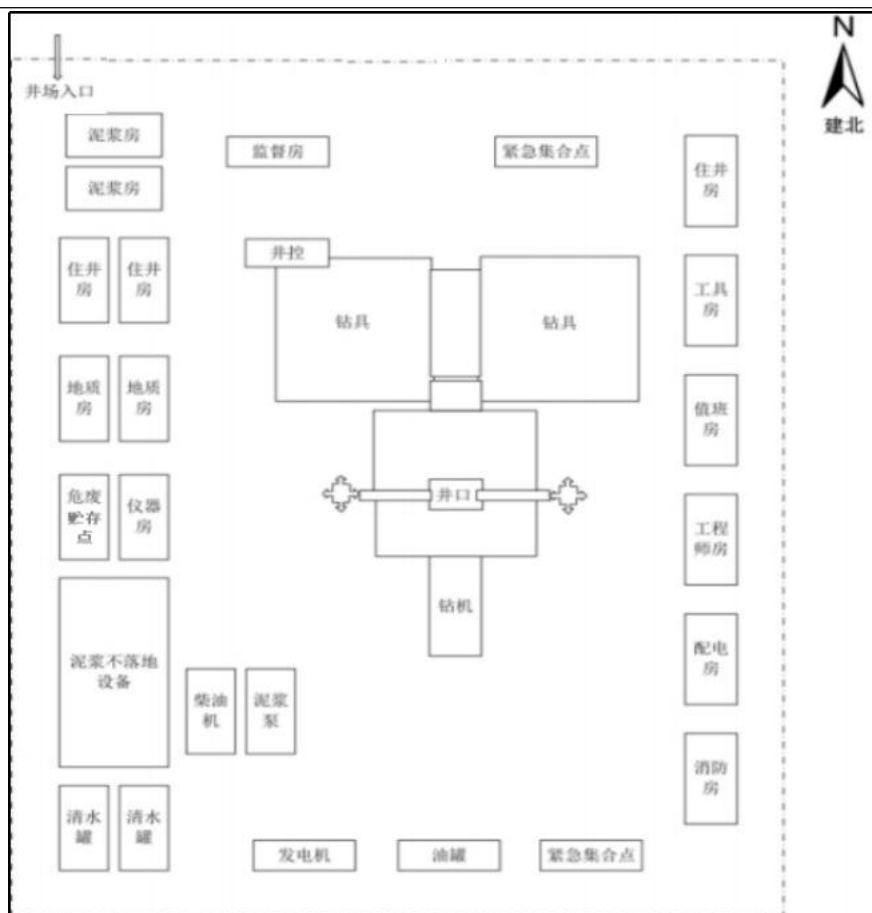
图 2-6 钻井井场平面布置示意图
