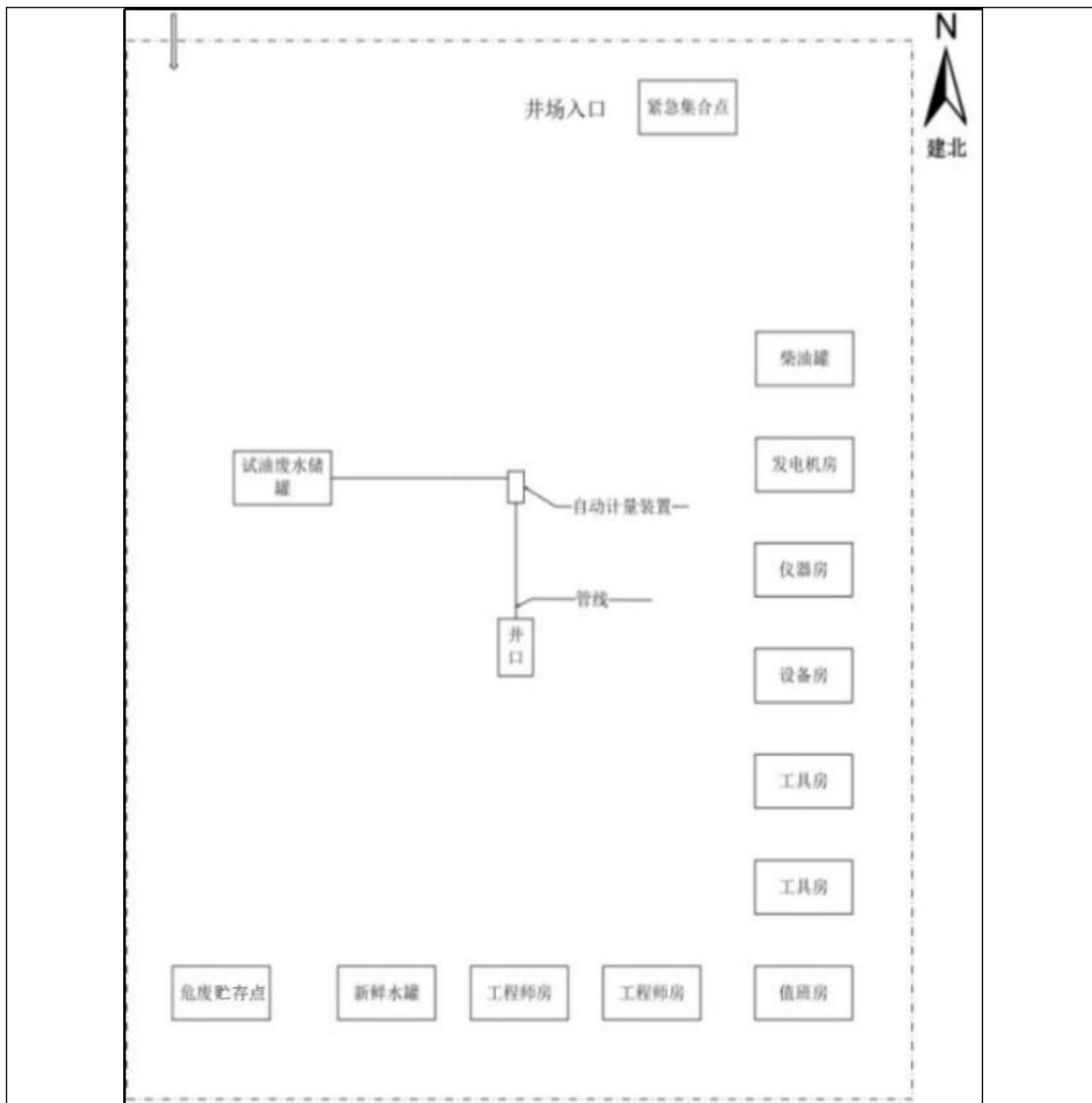
图 2-7 试油过程平面布置示意图
