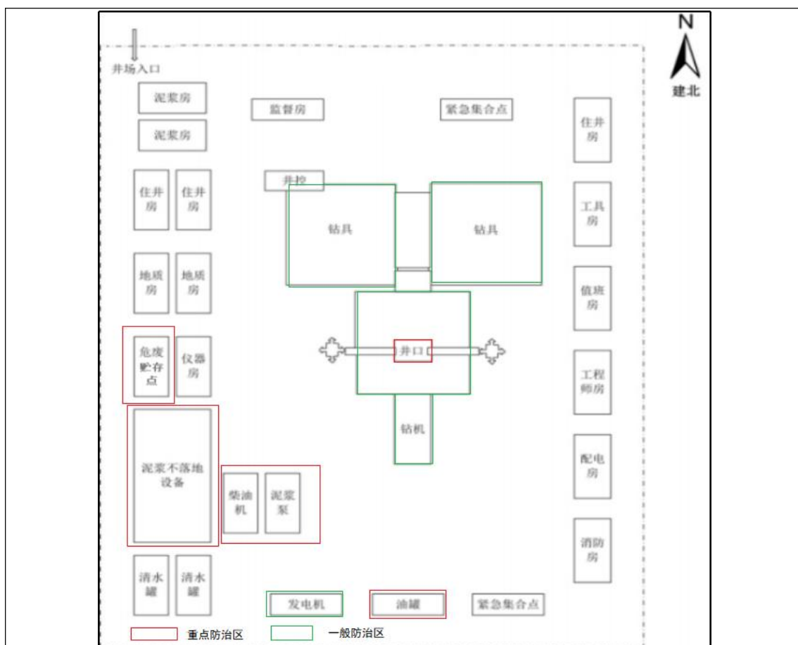
图 4-2 项目分区防渗图
