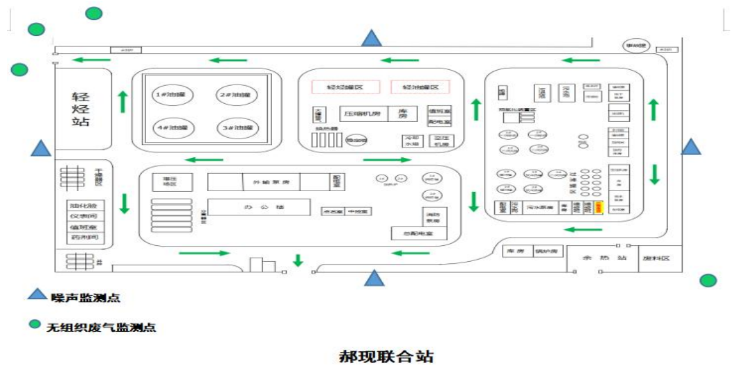
图 3 无组织废气监测点 (以郝现联为例, 根据实际风向调整, 上风向设 1 个参照点, 下风向设 3 个监控点)
