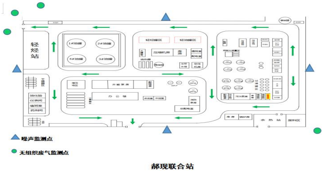
图 5 厂界噪声监测点位图（例）
