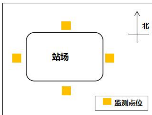
图 5 厂界噪声监测点位图
