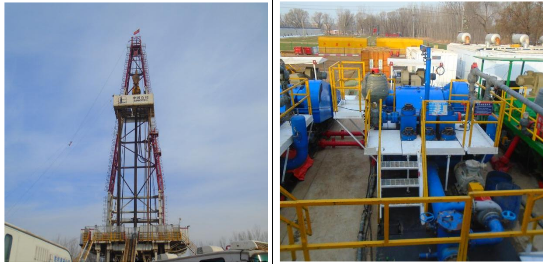
图 2-1 施工期现场照片
