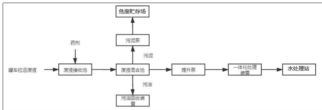
图 2-2 临盘废液处理站工艺流程示意图
