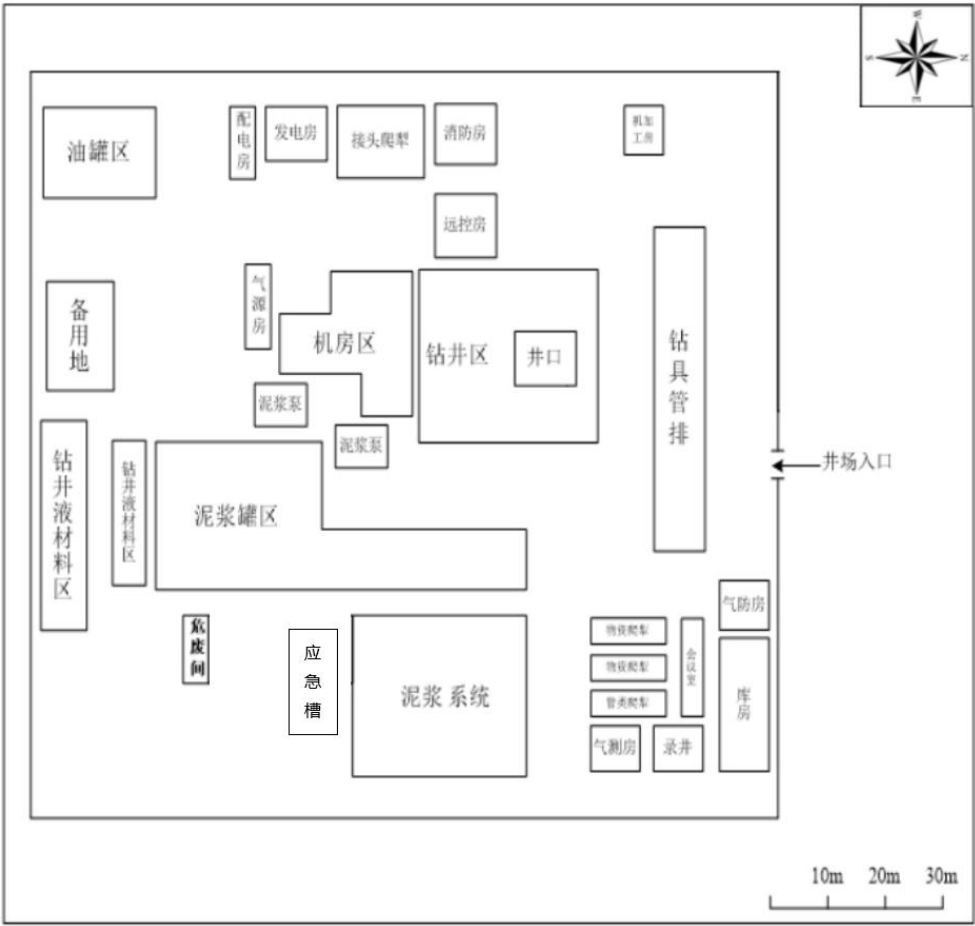
图 2-2 钻井井场布置示意图
