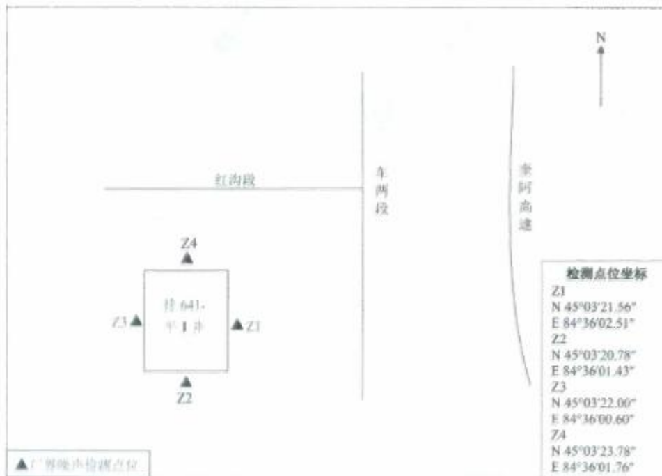
图 3-1 厂界噪声检测点位示意图
