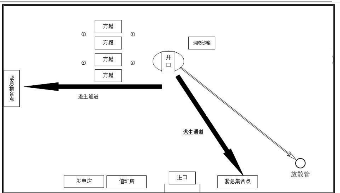
图 2-3 试油井场平面布置图
