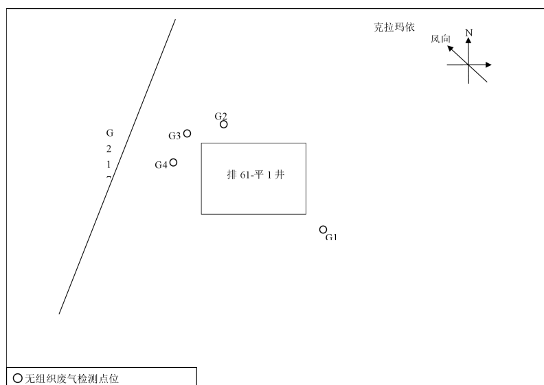
图 5 无组织废气监测点位示意图
