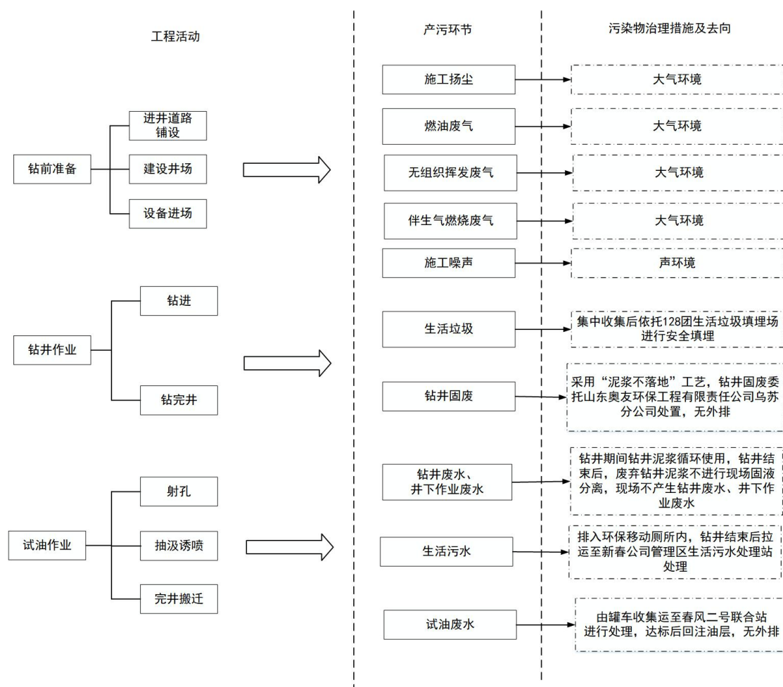
图 3 工艺流程及产污环节图
