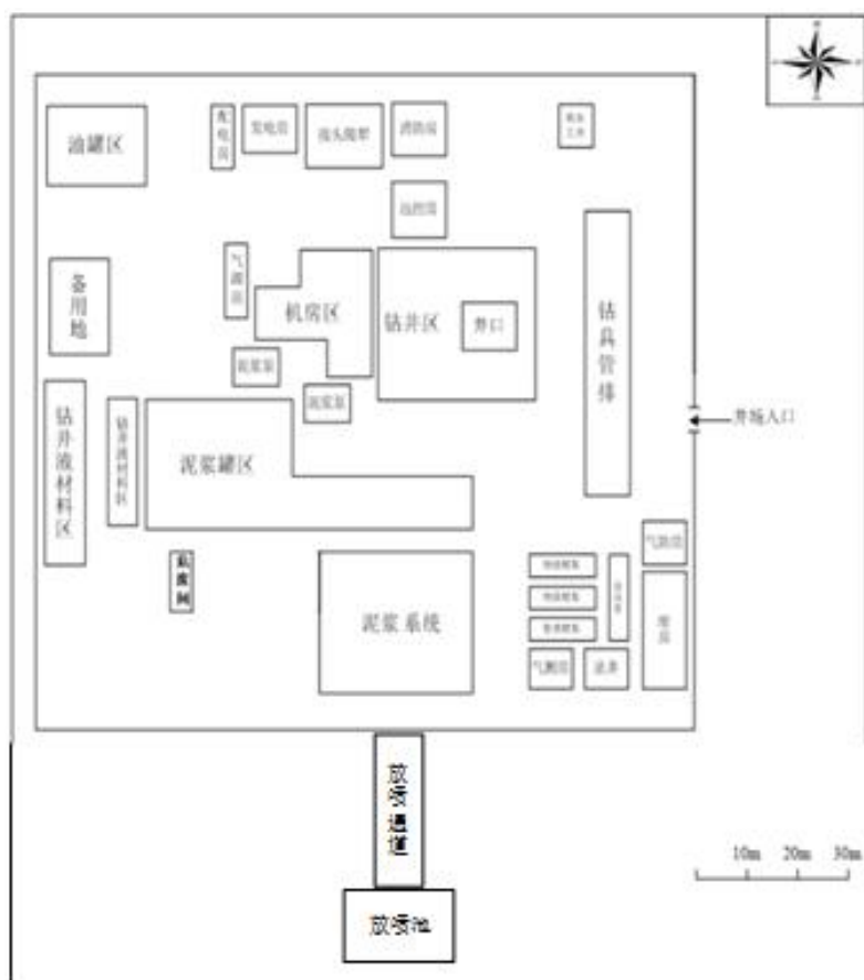
图 1 钻井工程平面布置图
