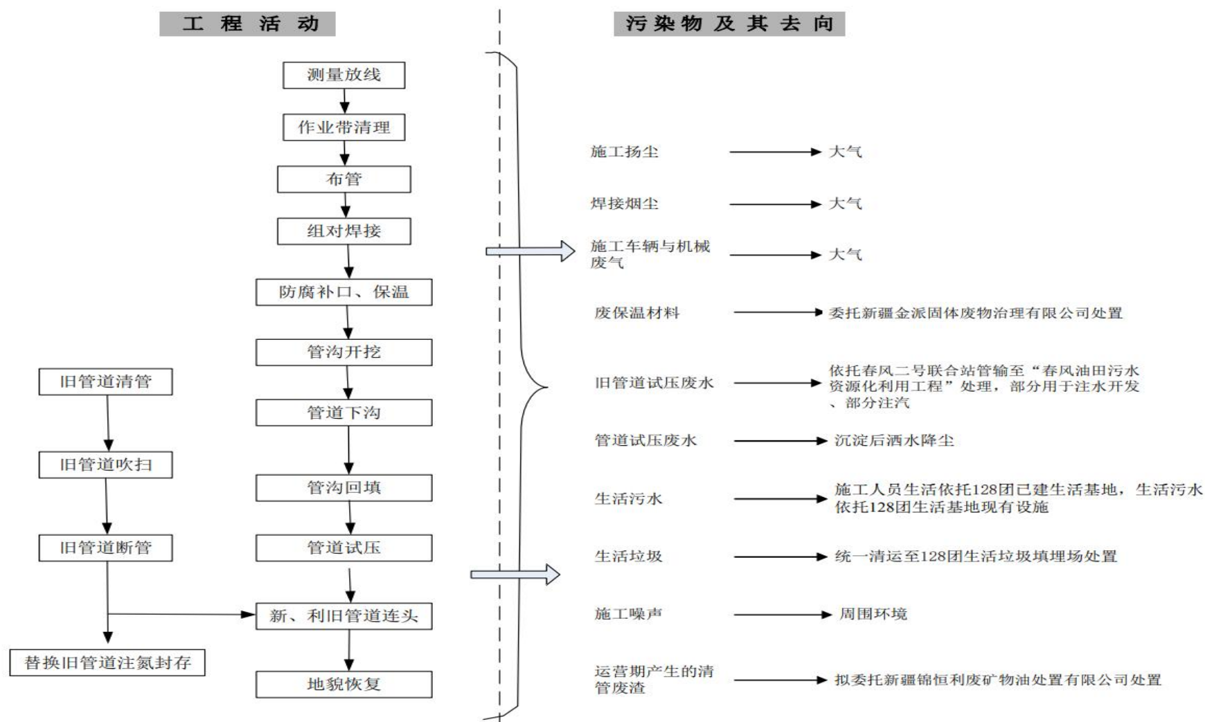
图 2- 5 施工工艺流程图及产污去向图
