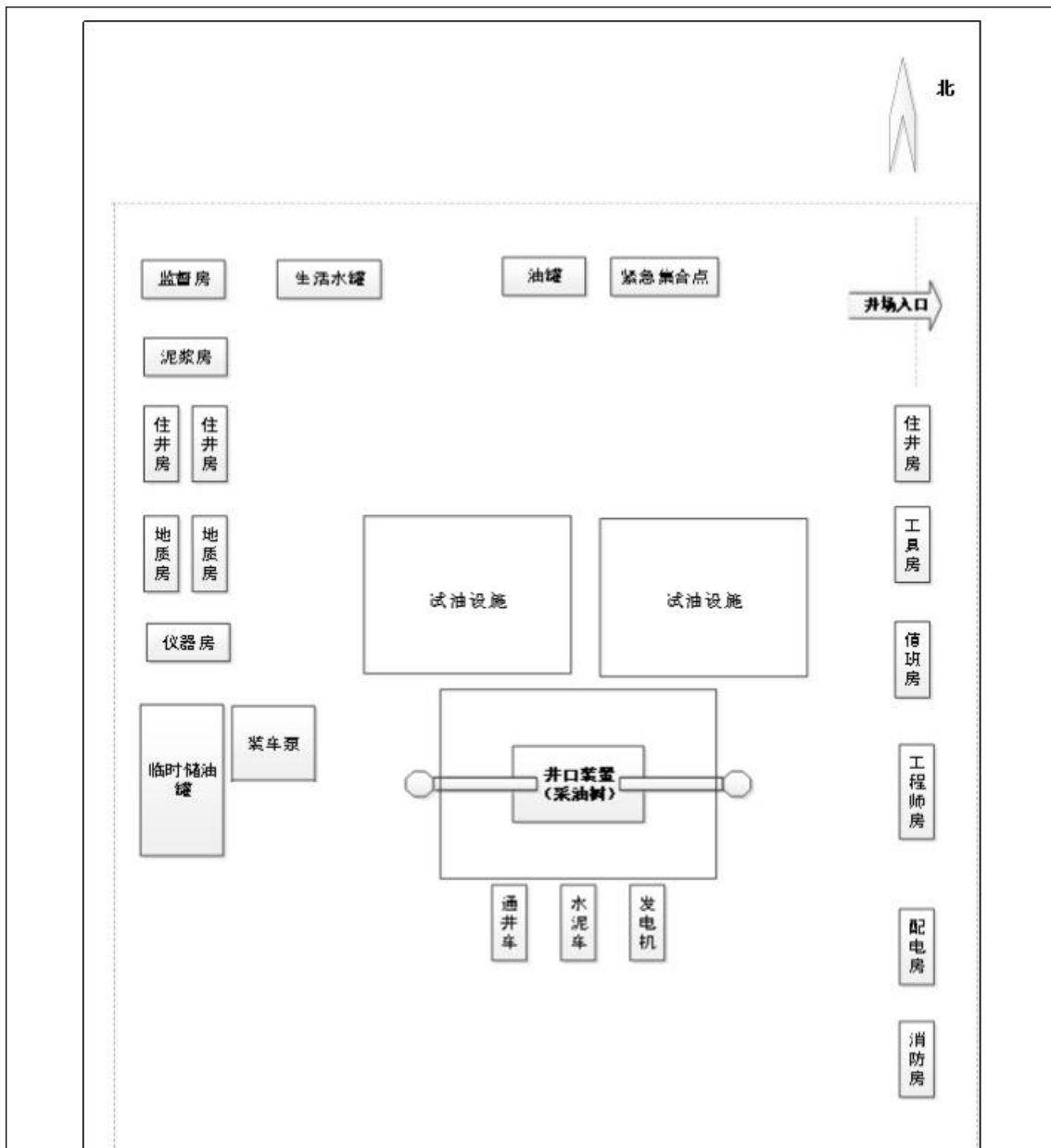
图 2-3 试油过程平面布置图
