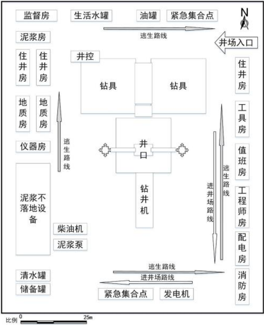
图 2-2 钻井井场平面布置示意图
