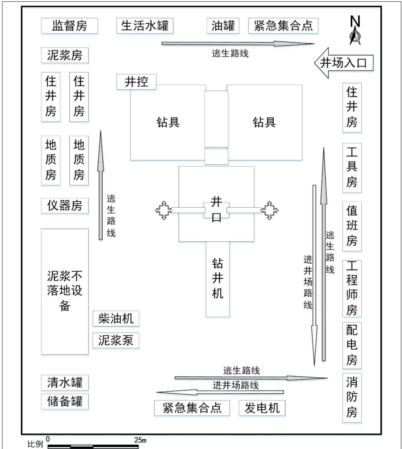
图 2-3 钻井与试油作业井场平面布置图
