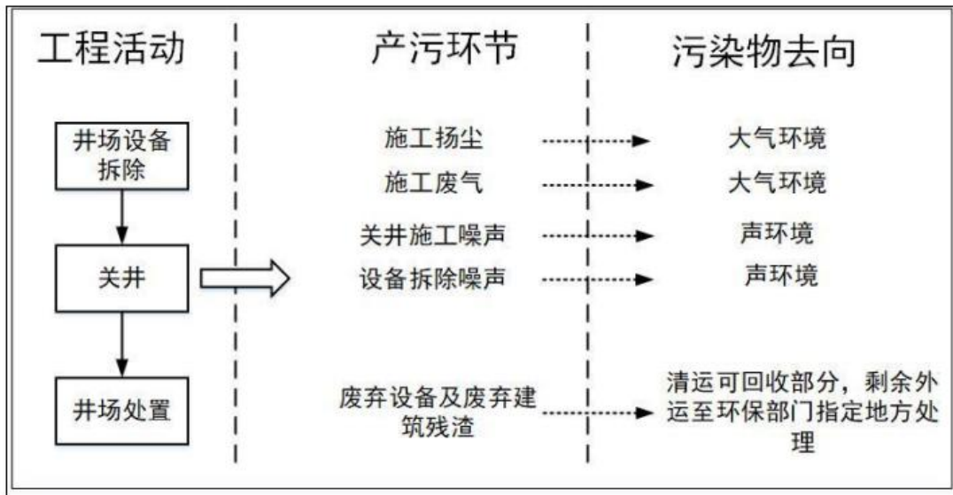
图 2-5 封井工艺流程及产污环节图
