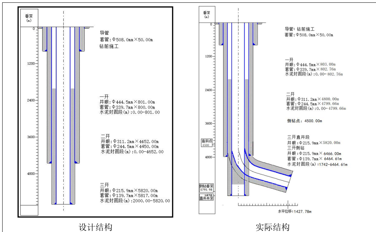
图 2-1 井身结构示意图
