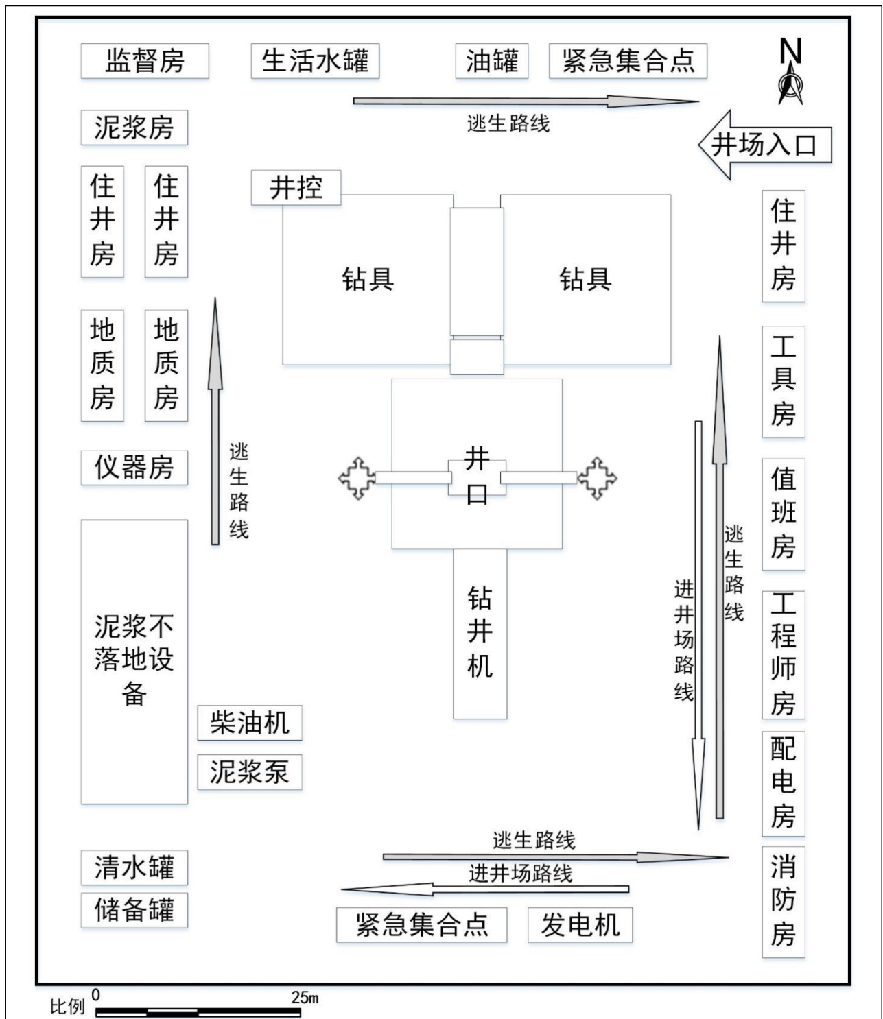
图 2-3 钻井及试油作业井场平面布置图
