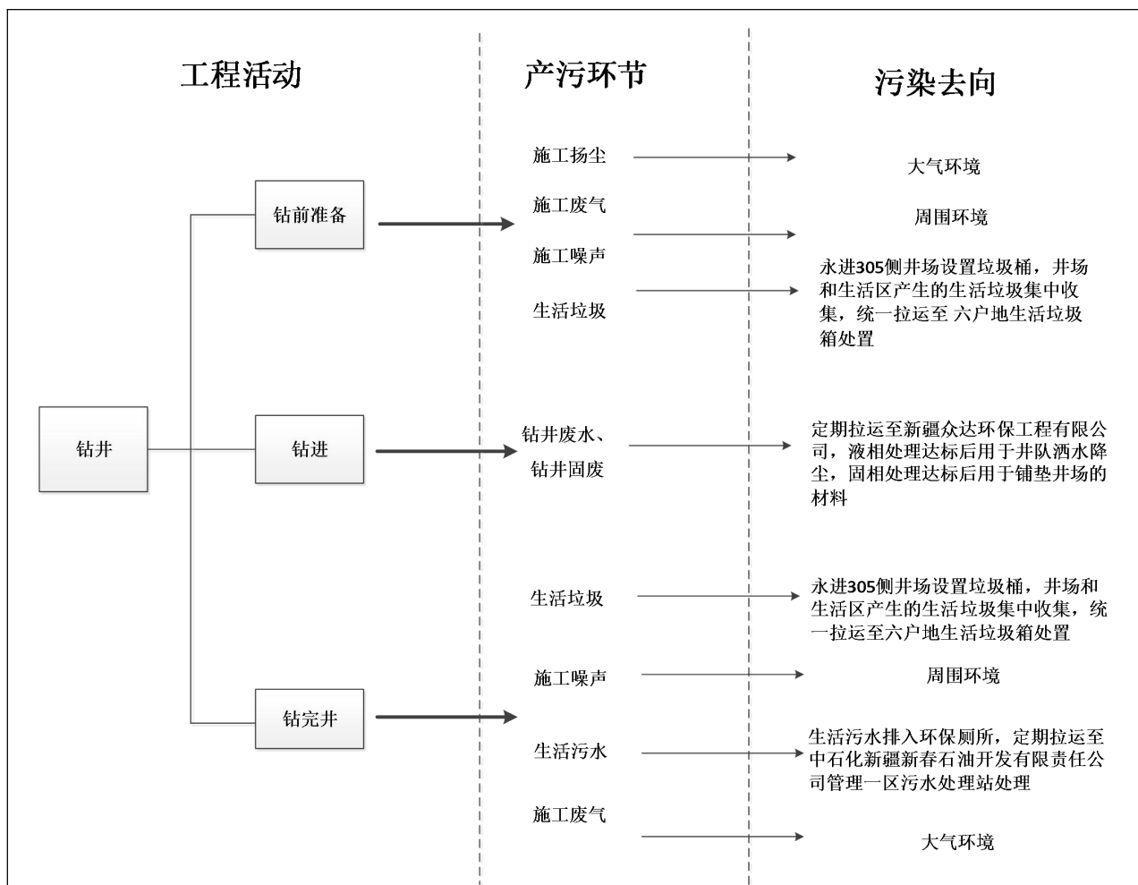
图 2-4 钻井和试油工艺流程及产污环节图
