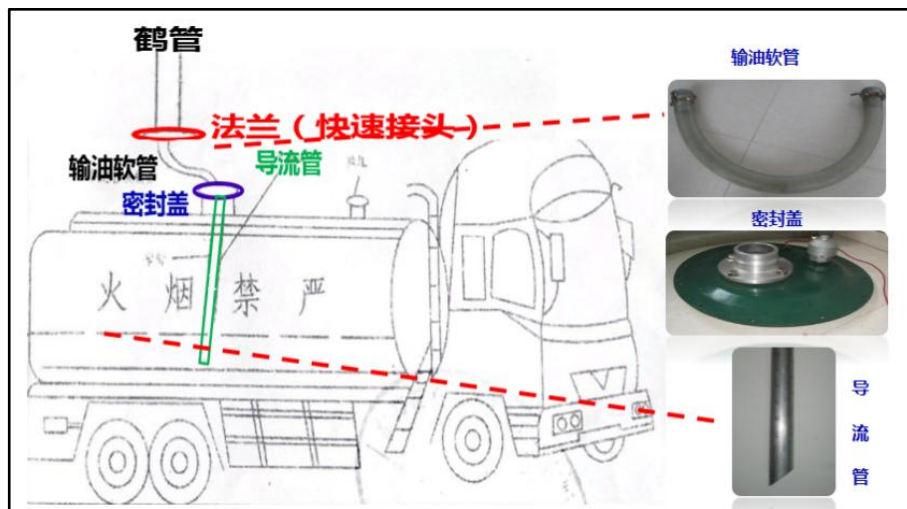
图 2-7 浸没式装车原理图
