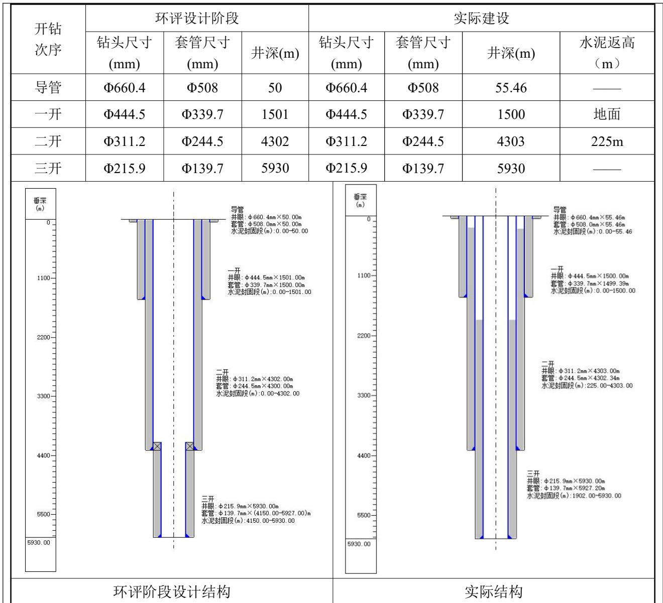
图 2-2 井身结构示意图
