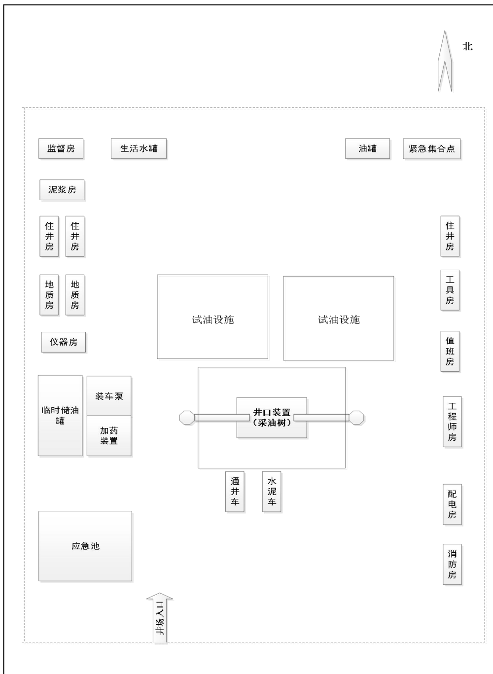
图 2-4 面布置
