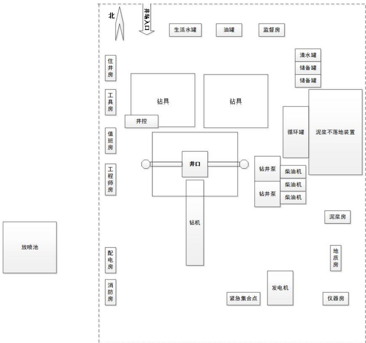
图 1 钻井井场平面布置图
