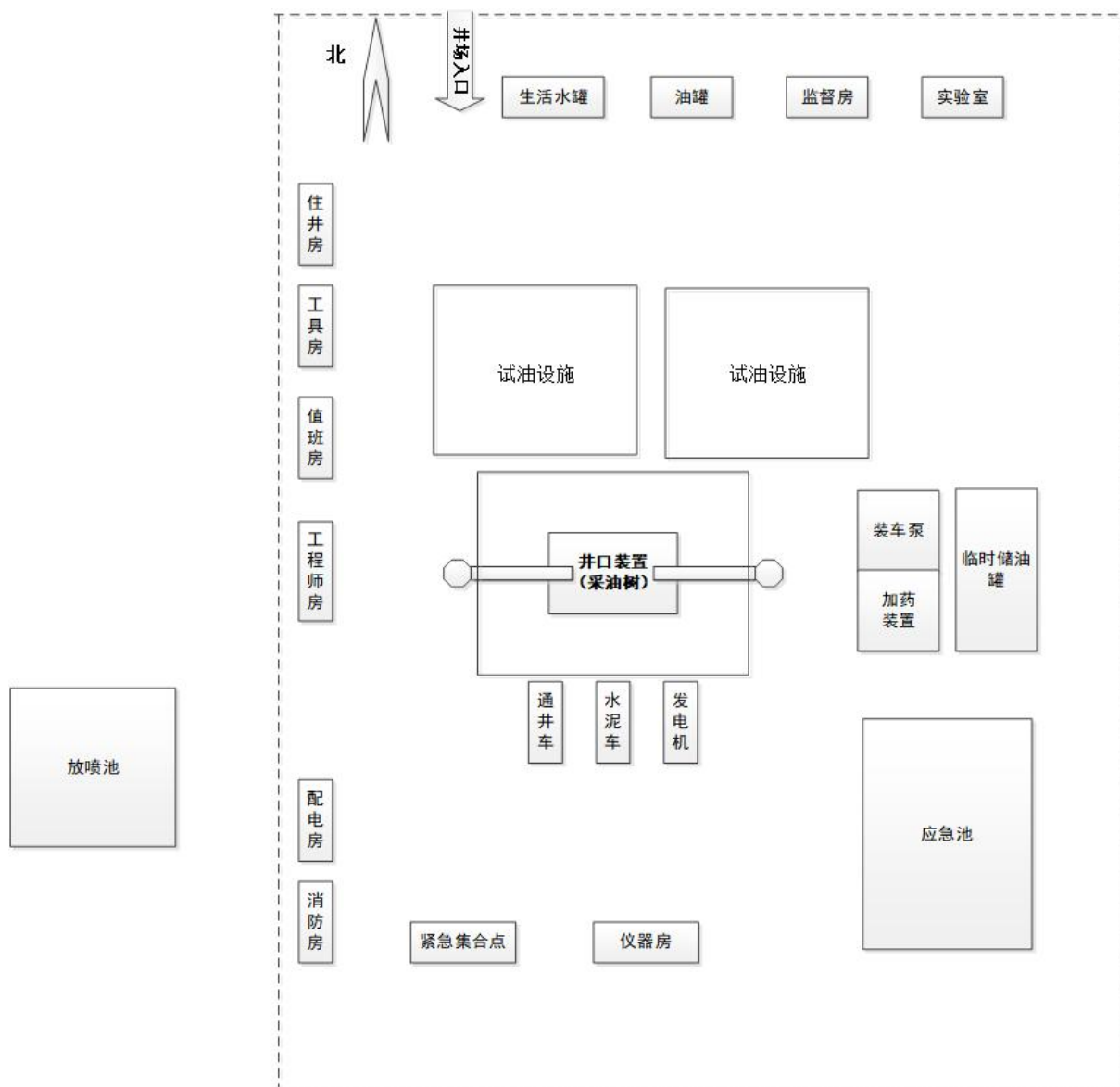
图 2 试油过程平面布置图
