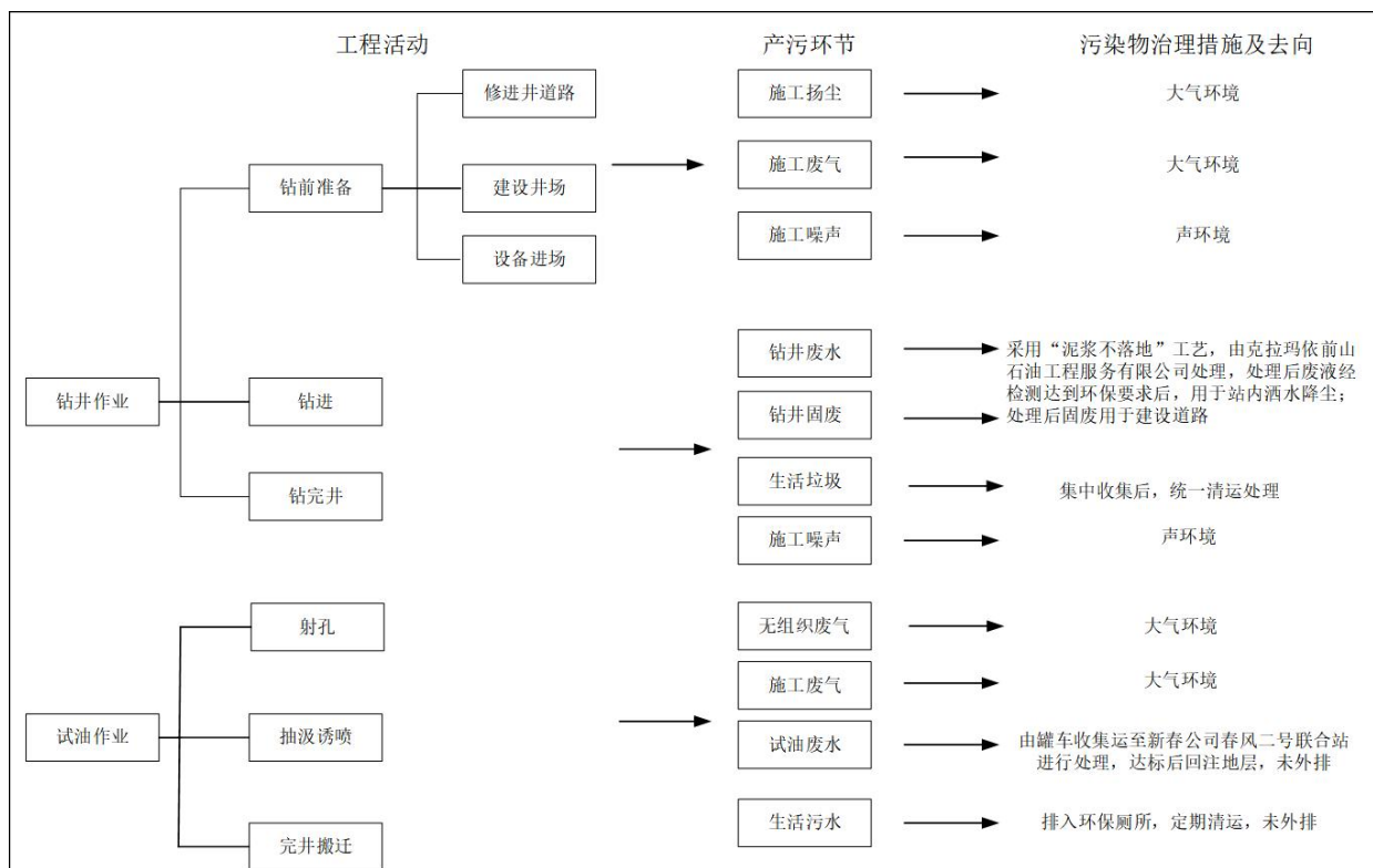
图 3 钻井及试油工艺流程及产污环节图
