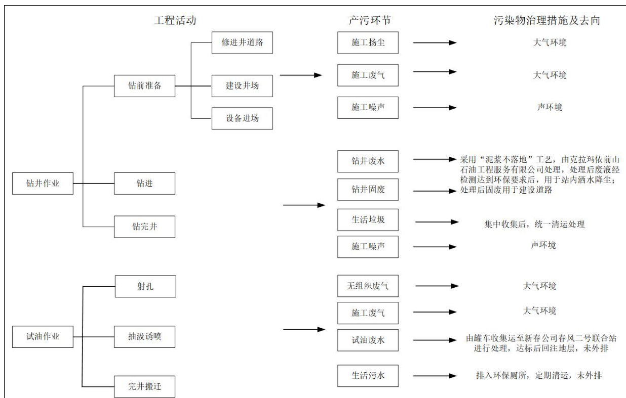
图 4 排 746 井钻井及试油工艺流程及产污环节图
