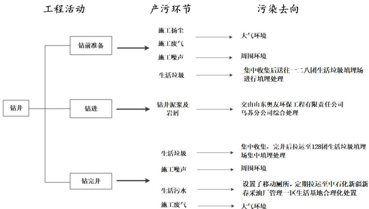
图 5 排 747、748 井钻井及试油工艺流程及产污环节图
