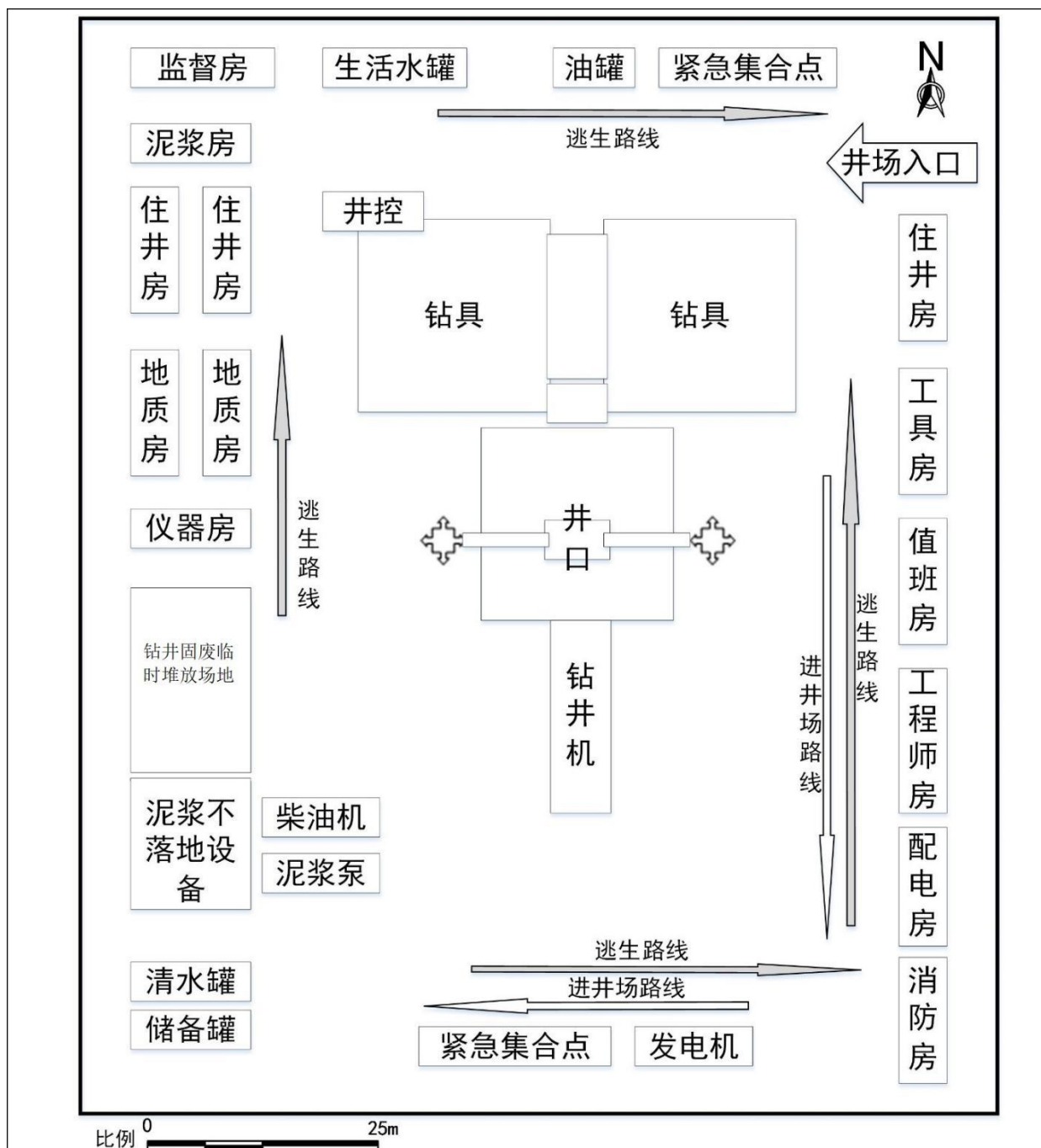
图 3 钻井作业井场平面布置示意图
