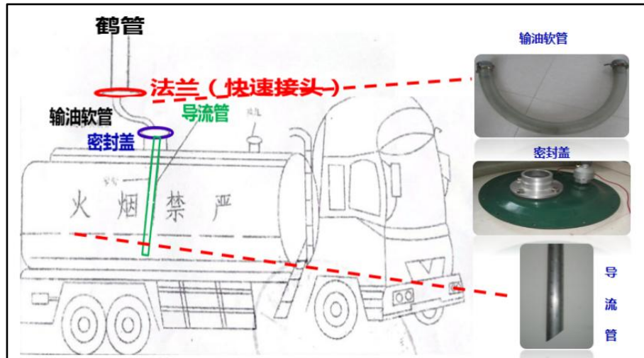
图 7 浸没式装车原理图
