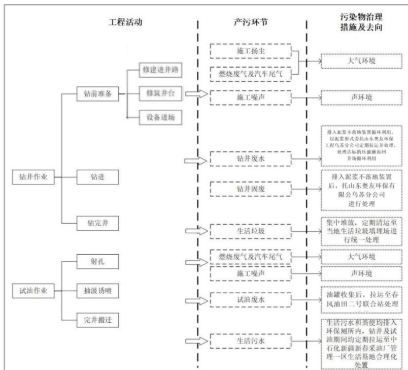
图 2-4 钻井和试油工艺流程及产污环节图
