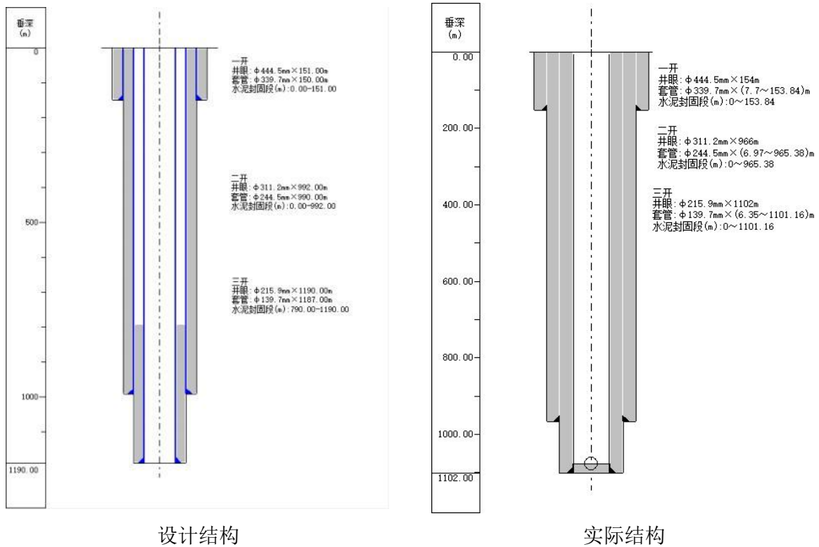
图 2-1 井身结构示意图
