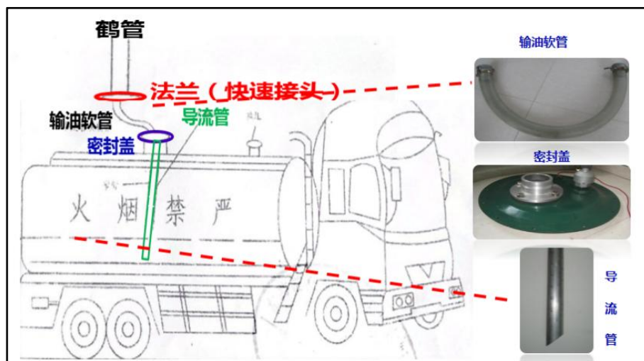
图 2-6 浸没式装车原理图
