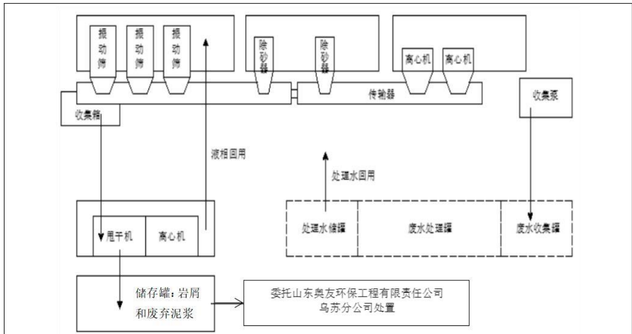
图 2-5 泥浆不落地工艺流程示意图
