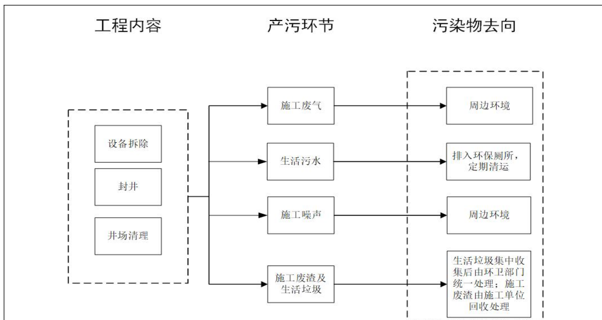
图 2-6 封井工艺流程及产污环节图
