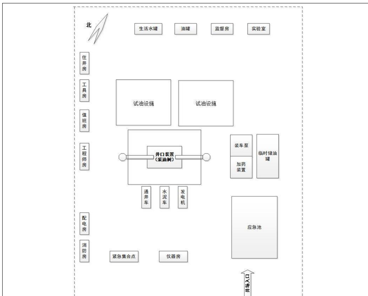
图 2-3 试油作业井场平面布置图
