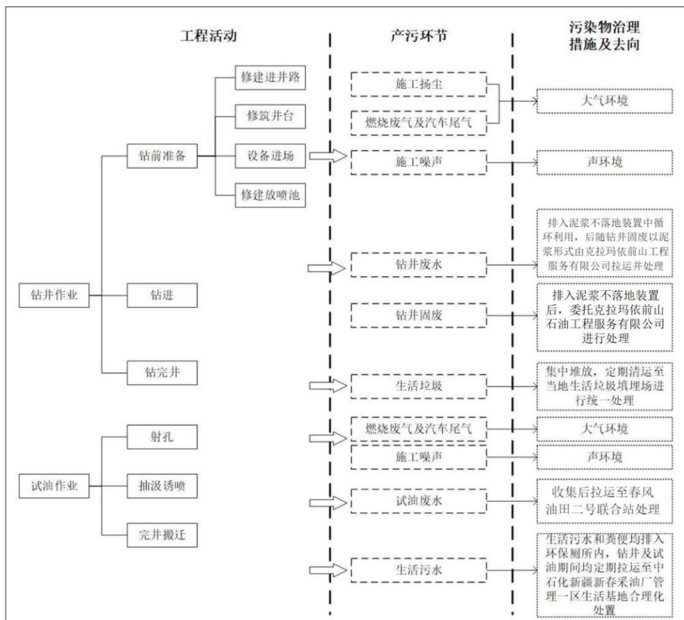
图 2-4 钻井和试油工艺流程及产污环节图
