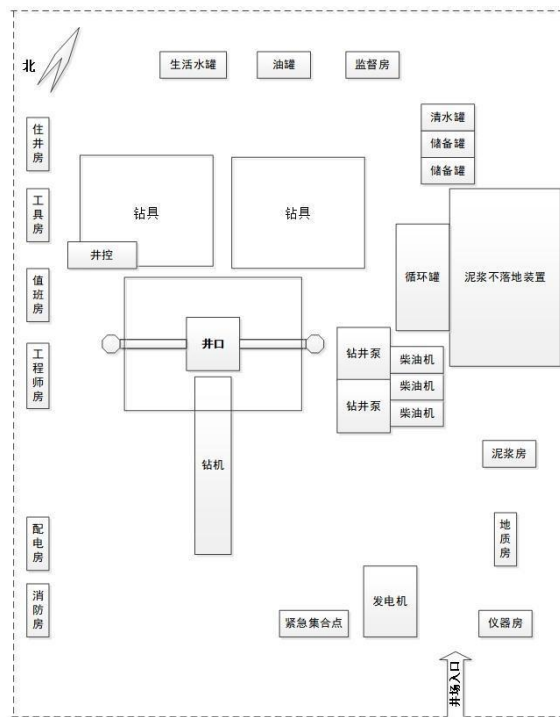
图 2-2 钻井作业井场平面布置图
