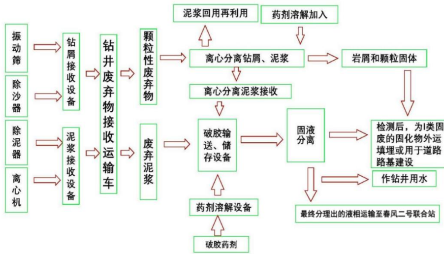
图 2-5 泥浆不落地工艺流程图
