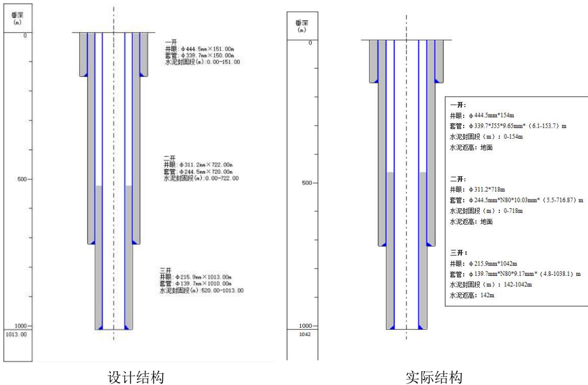
图 2-1 井身结构示意图
