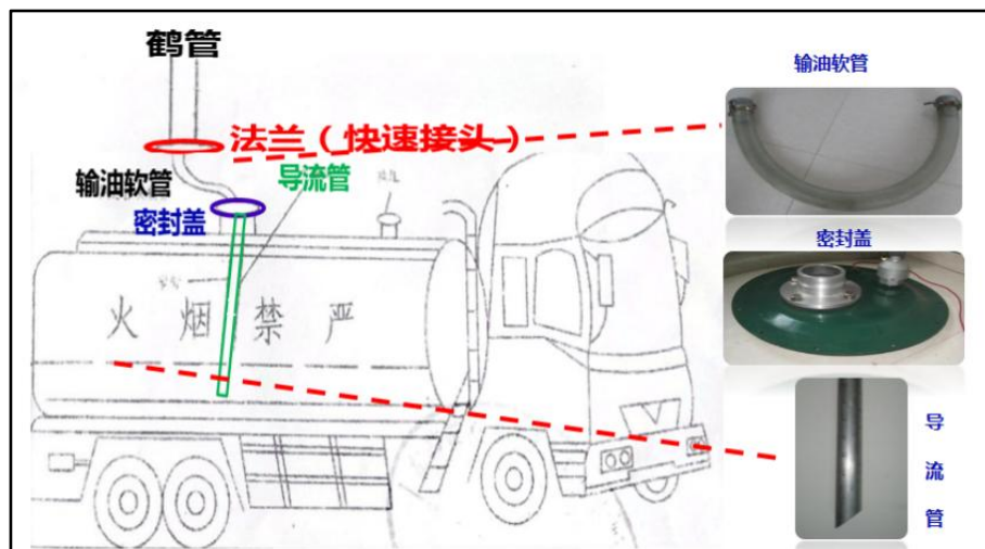
图 2-7 浸没式装车原理图
