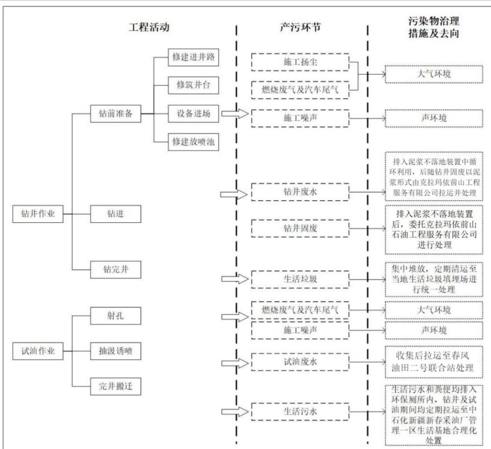
图 2-5 钻井和试油工艺流程及产污环节图
