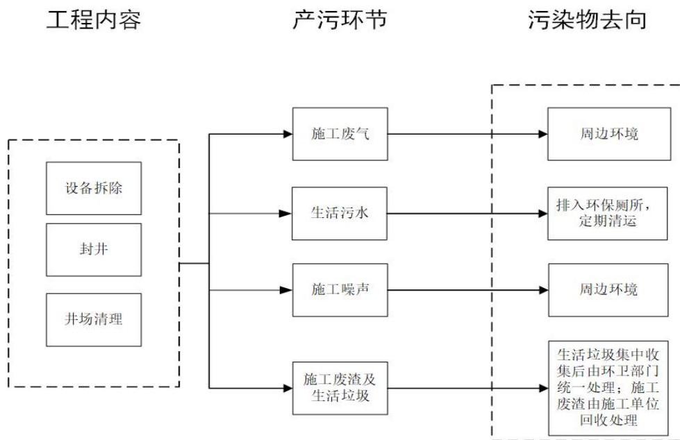
图 2-7 封井工艺流程及产污环节图
