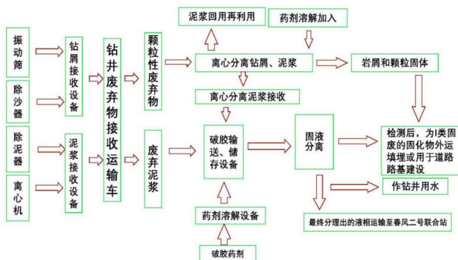
图 2-6 泥浆不落地工艺流程图
