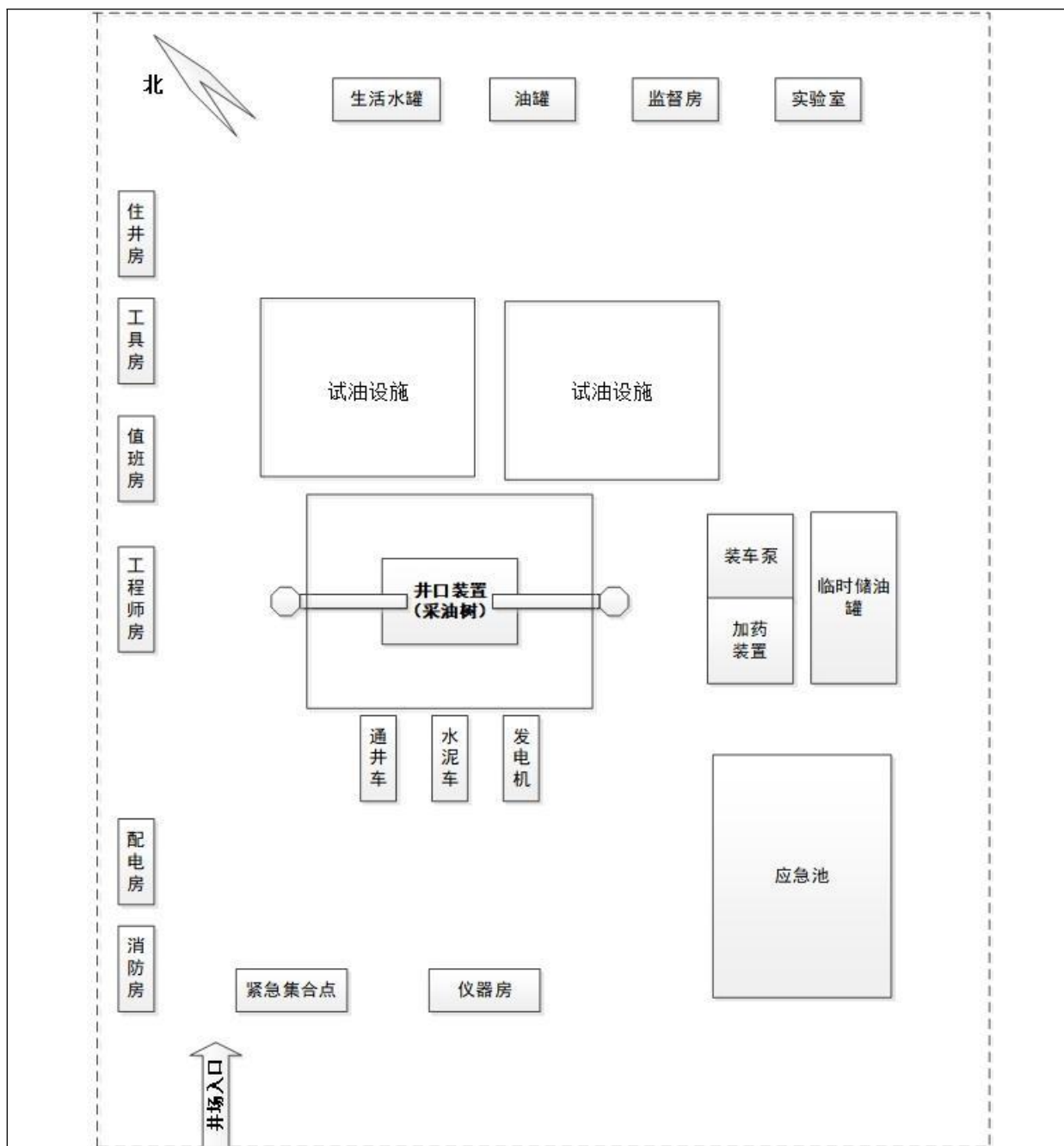
图 2-4 试油作业井场平面布置图
