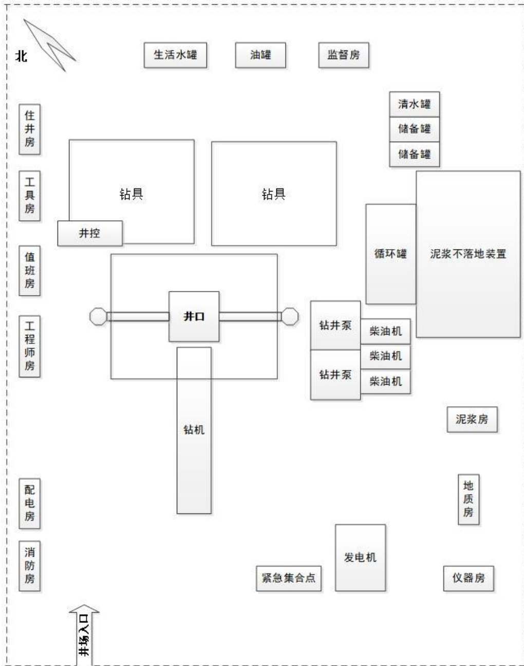
图 2-3 钻井作业井场平面布置图
