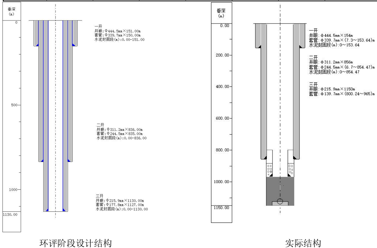
图 2-1 井身结构示意图
