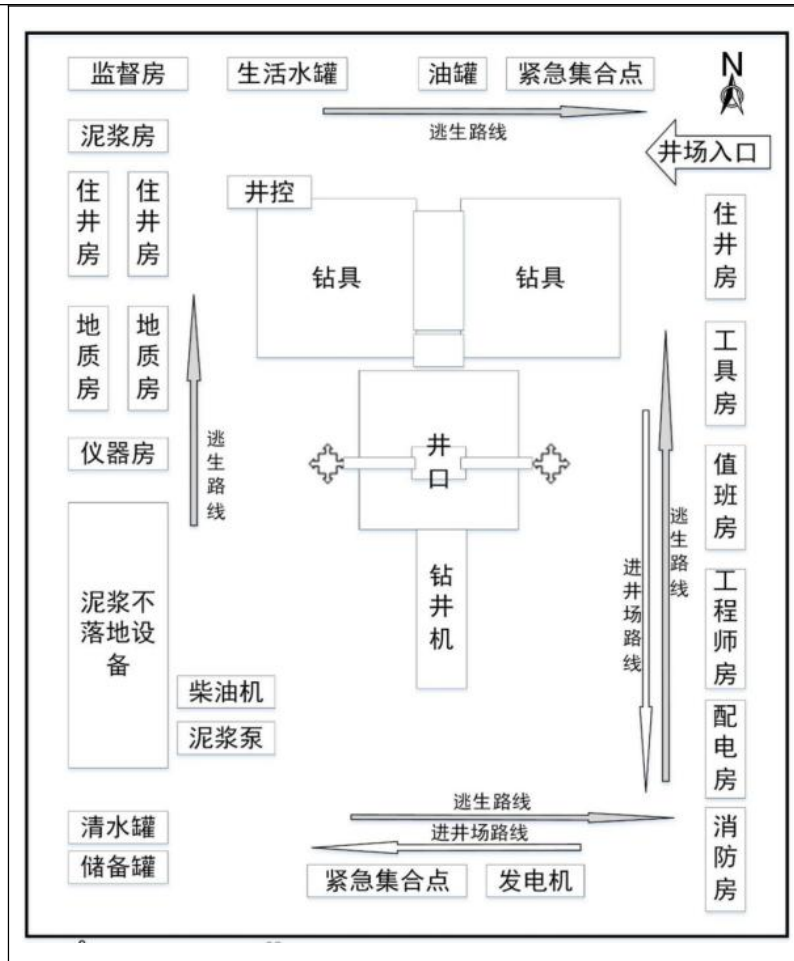
图 2-3 钻井与试油作业井场平面布置示意图
