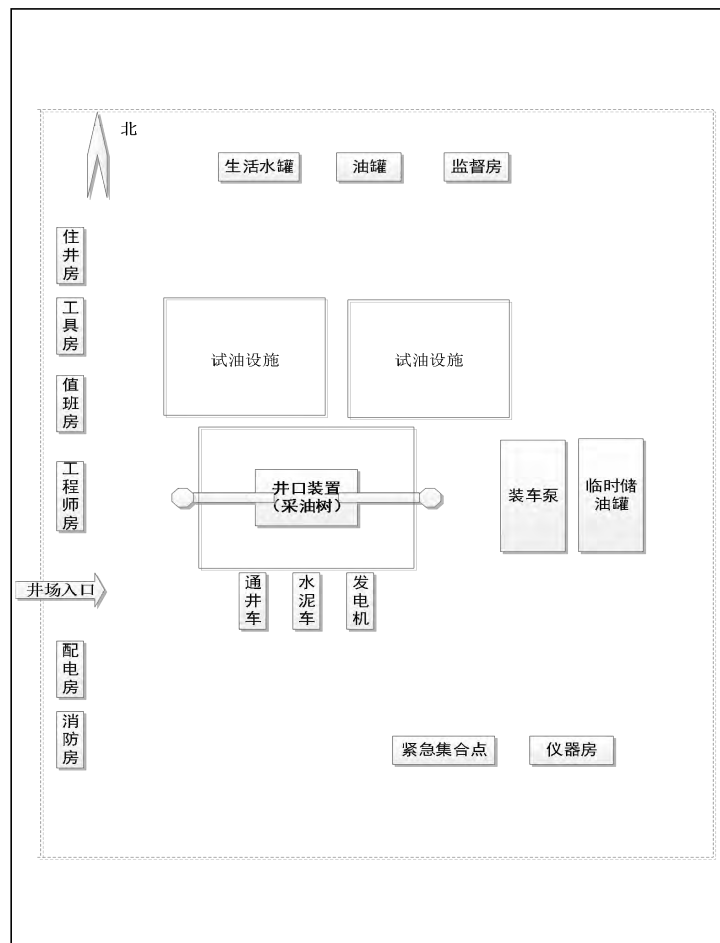
图 2-2 试油过程平面布置图
