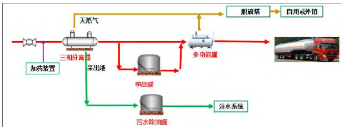
图 2-1 官七接转站工艺流程示意图
