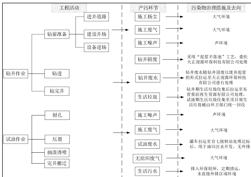
图 2-3 钻井及试油工艺流程及产污环节图
