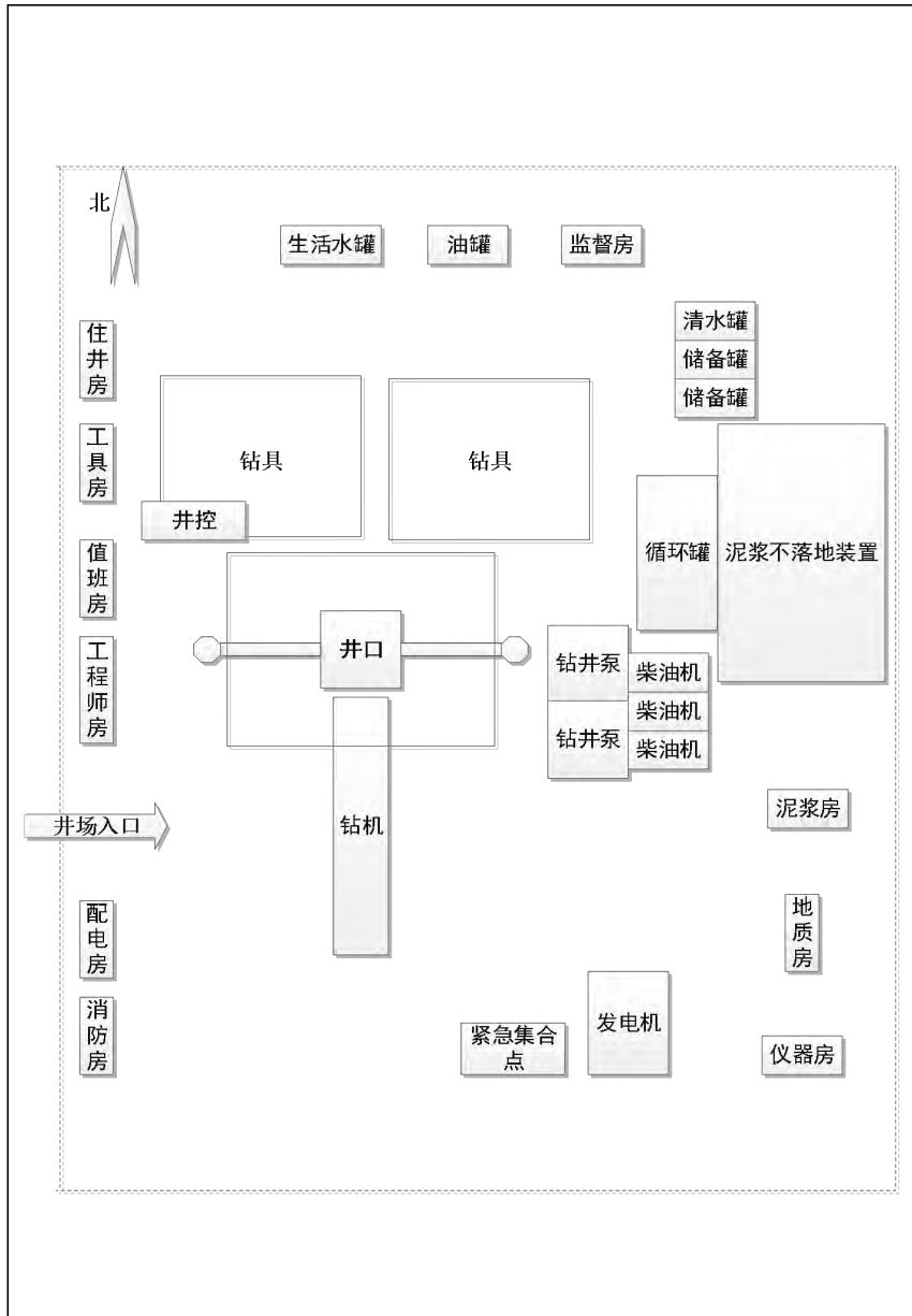
图 2-1 钻井井场平面布置图
