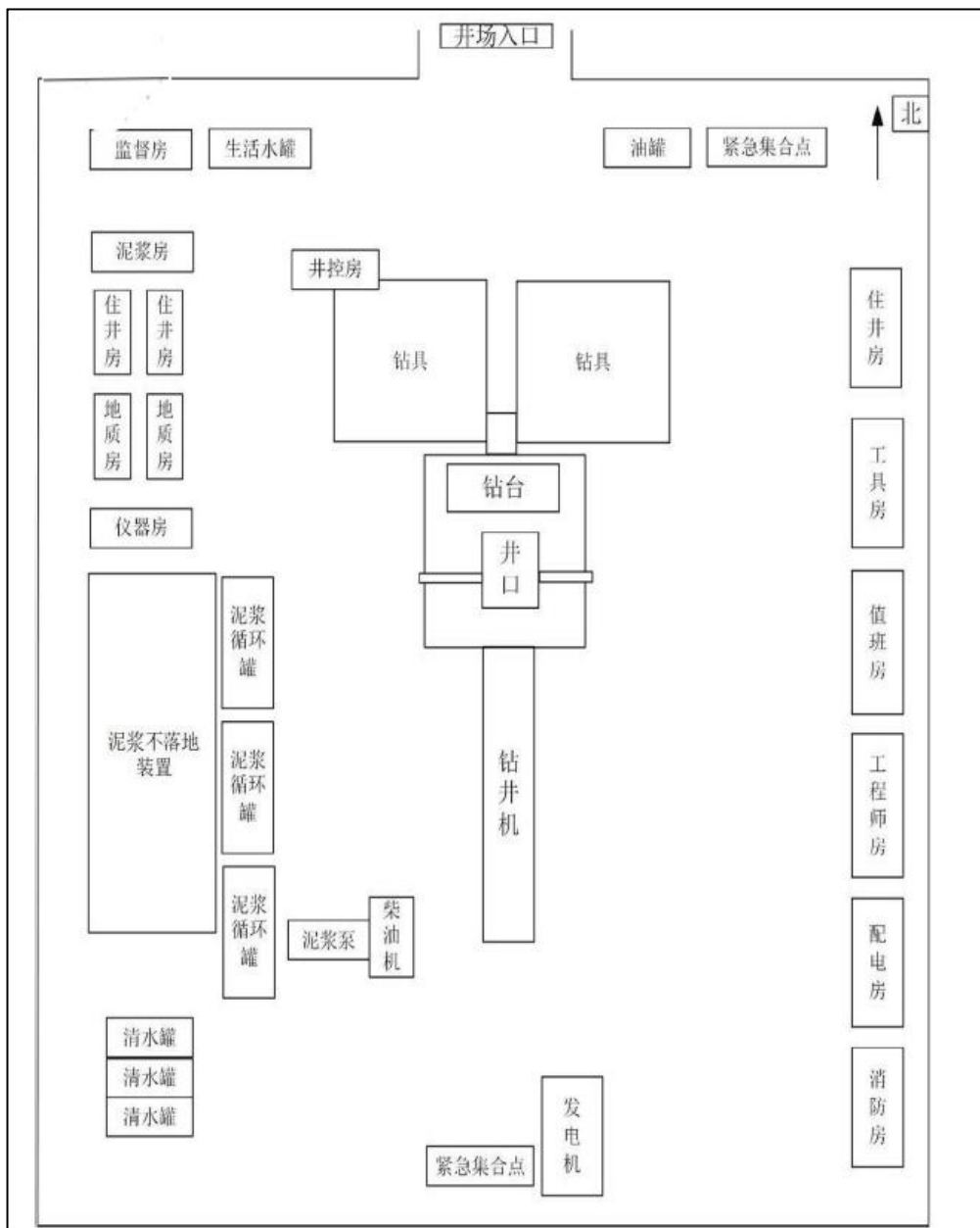
图 2-2 钻井井场平面布置示意图
