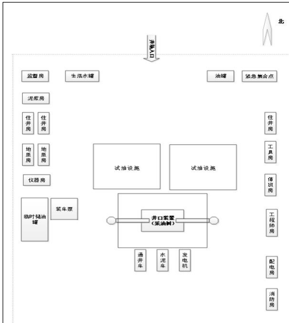
图 2-3 试油过程平面布置图
