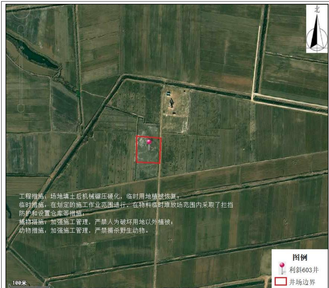
图 2-7 生态保护工程平面布置图
