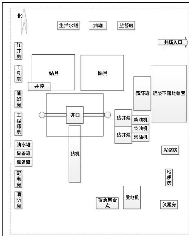
图 2-3 钻井井场平面布置示意图
