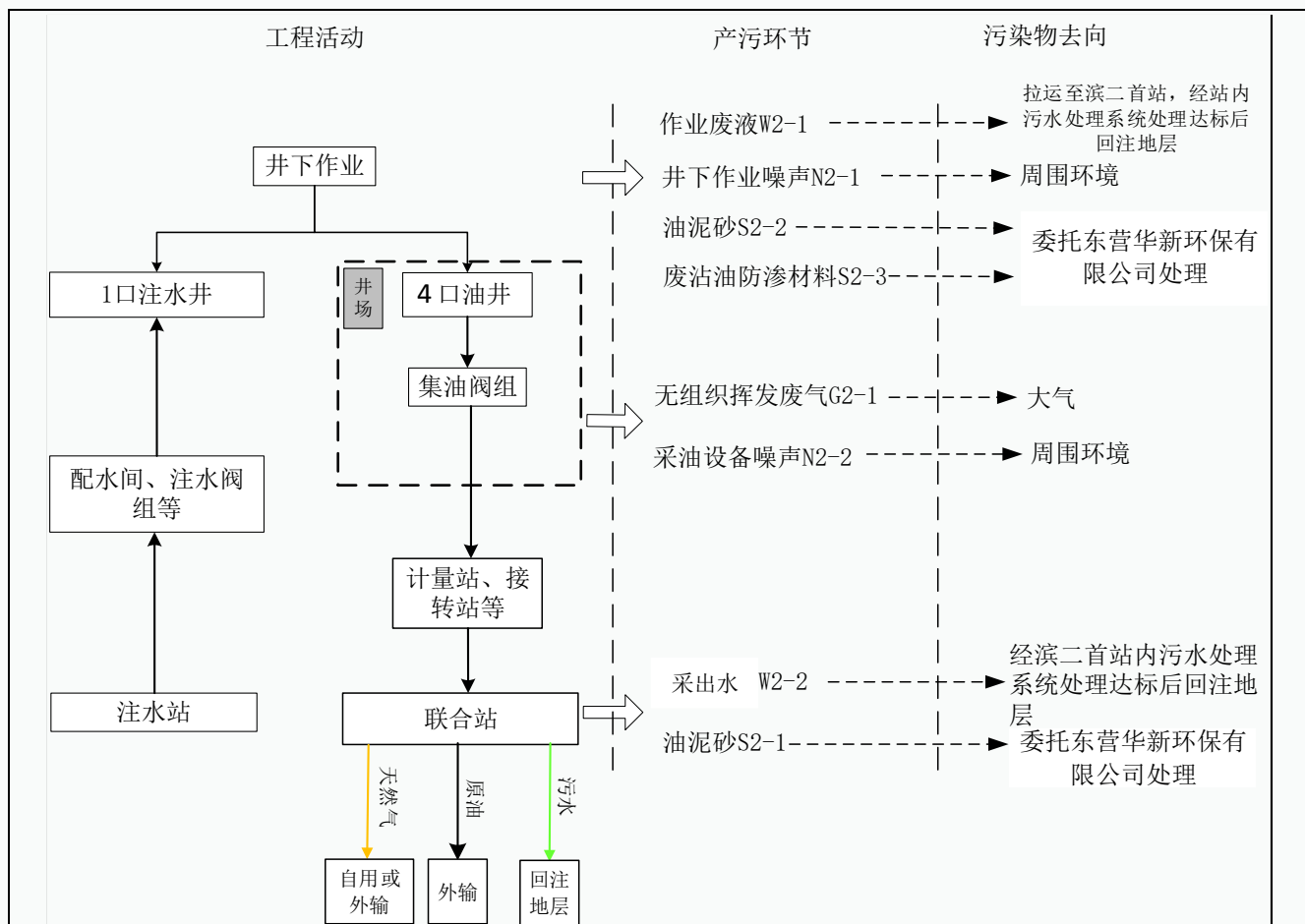
图 2-5 运营期工艺流程及主要产污环节图
