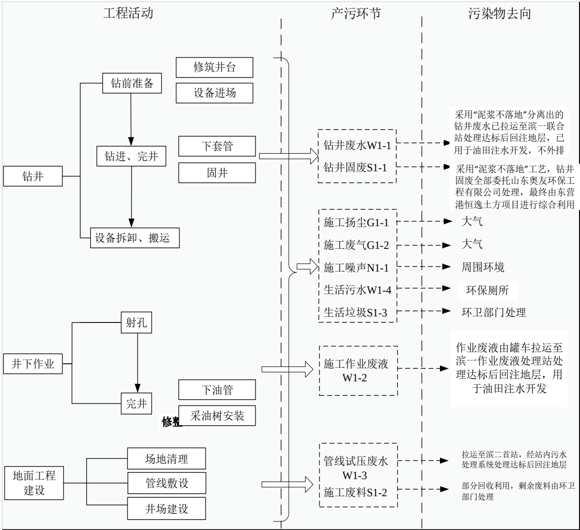
图 2-4 施工期主要工艺流程及产排污情况
