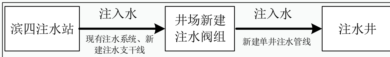
图 2-2 本项目注水流程示意图
