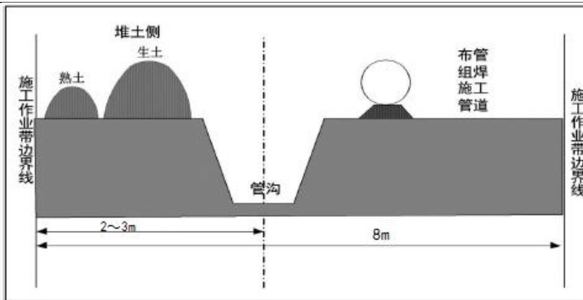
图 2-3 大开挖施工方式断面示意图
