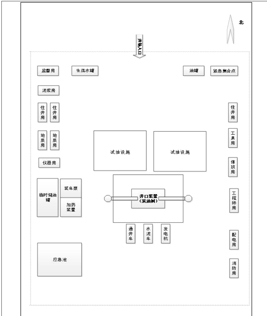
图 2-3 试油过程平面布置图
