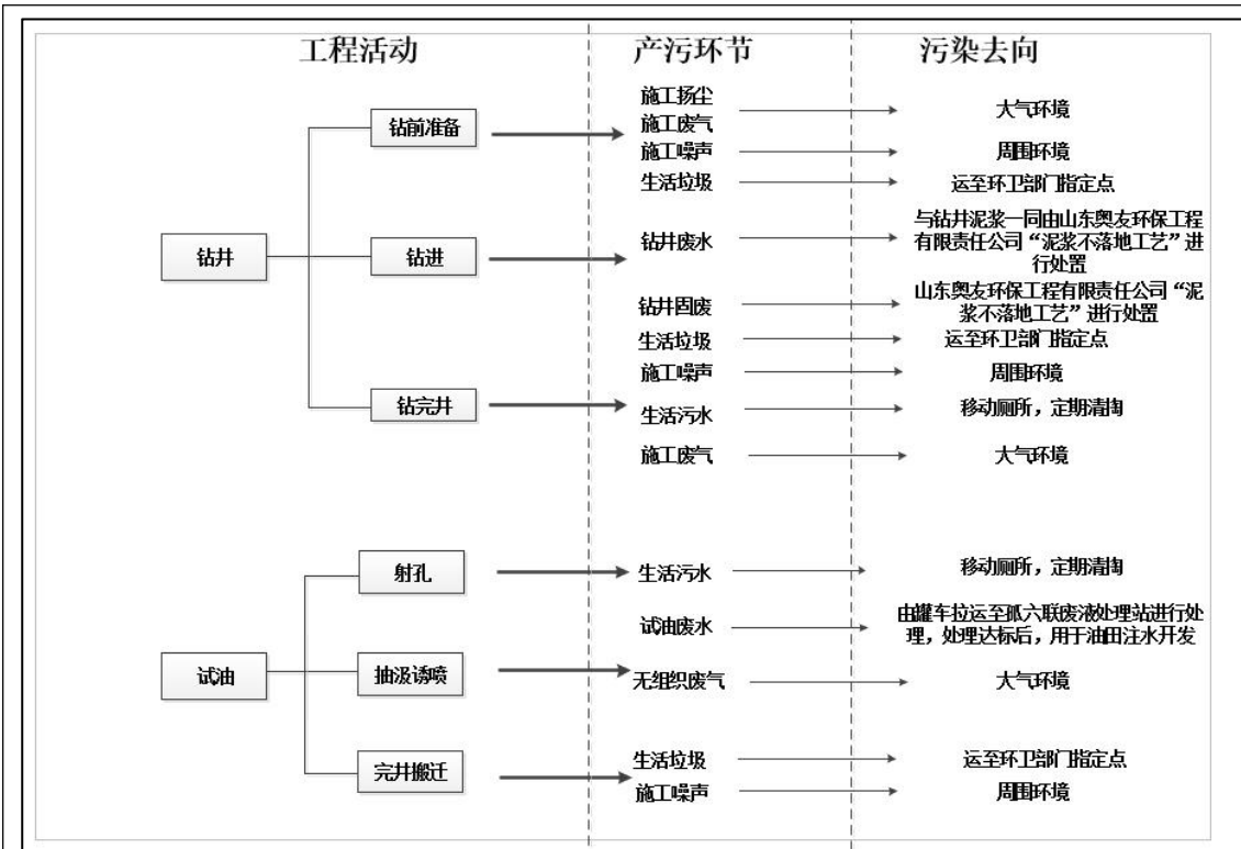
图 2-4 钻井及试油工艺流程及产污环节图
