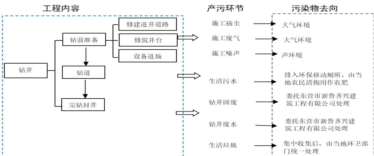
图 3 钻井工艺流程及产污环节图
