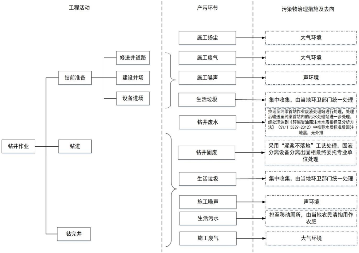
图 3 钻井工艺流程及产污环节图
