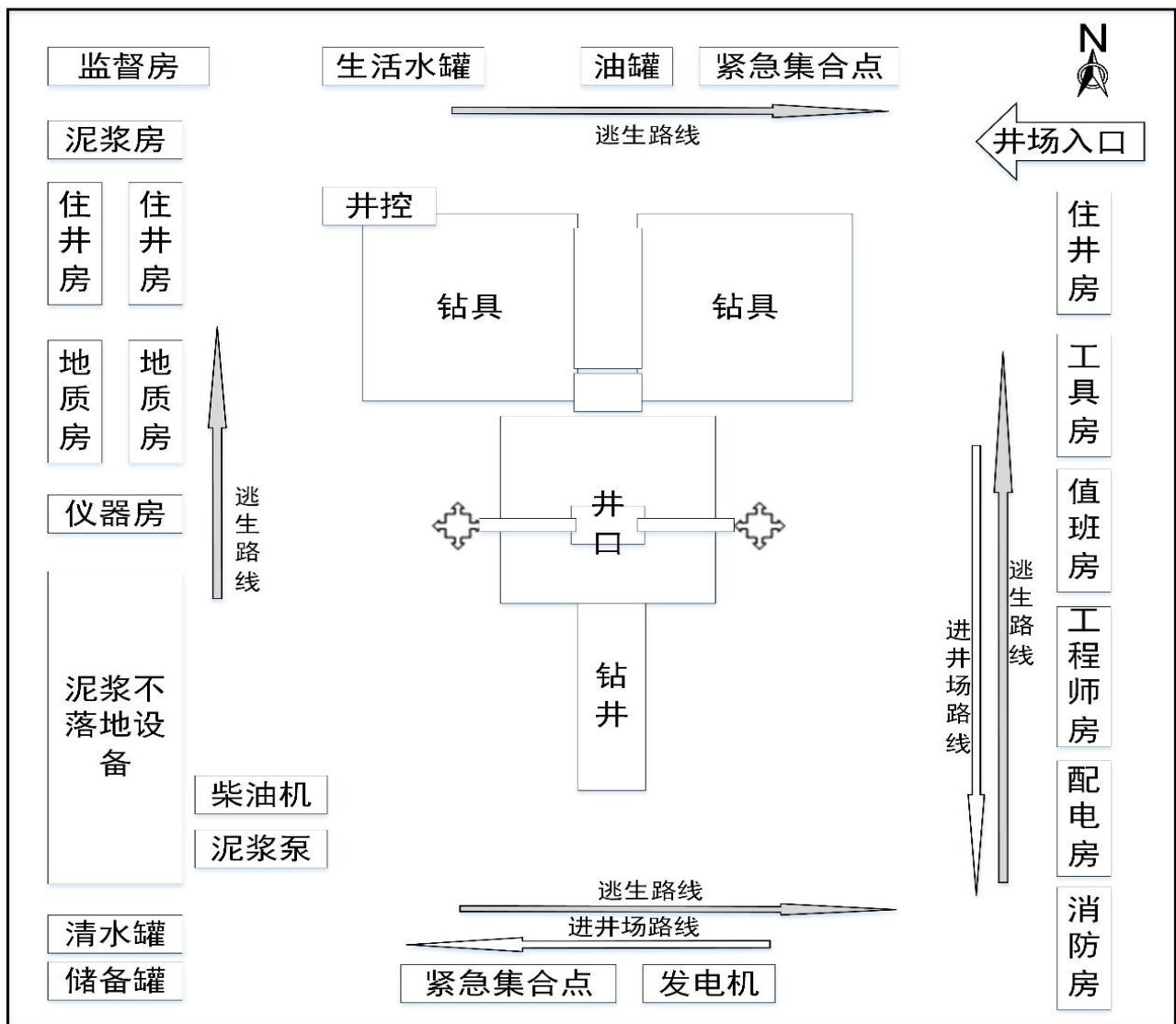
图 2 钻井井场平面布置示意图
