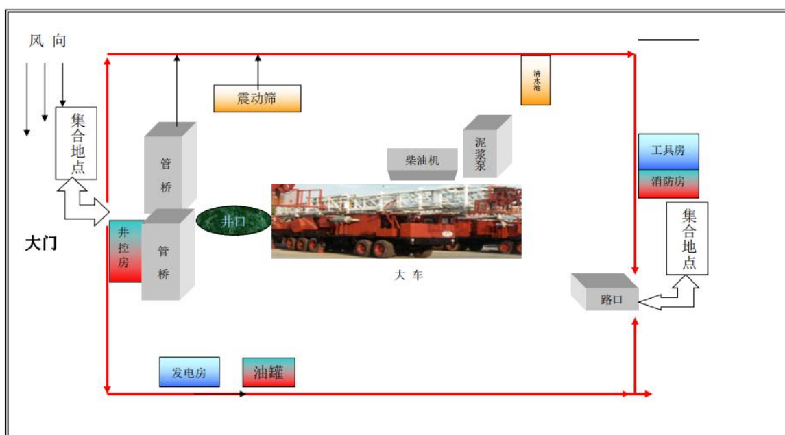
图 2-3 钻井井场平面图
