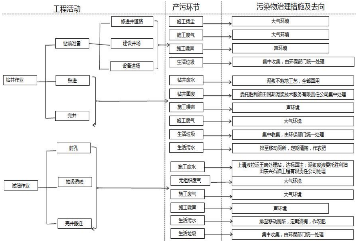
图 2-4 钻井及试油工艺流程及产污环节图
