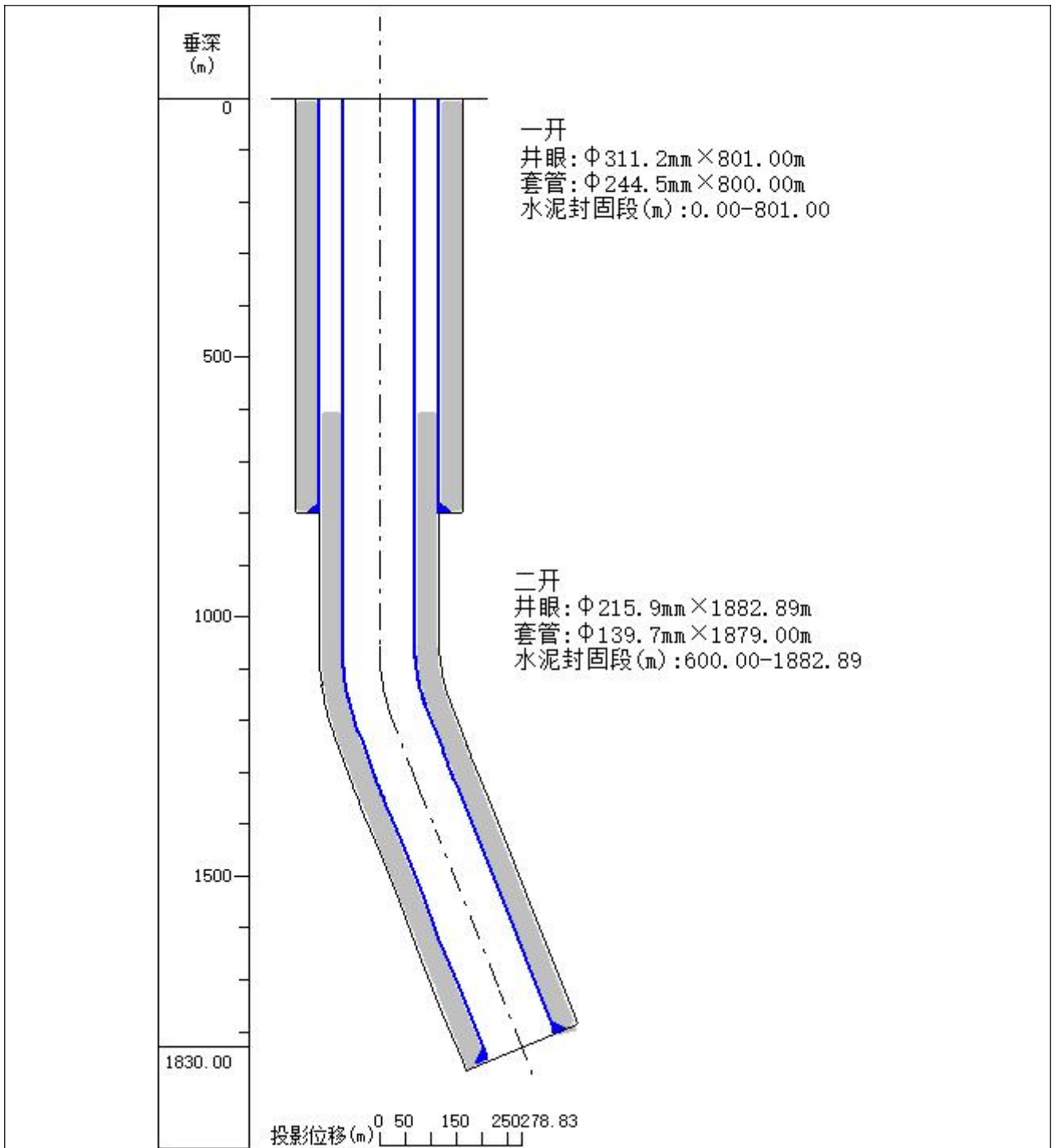
图 2-1 井深结构示意图
