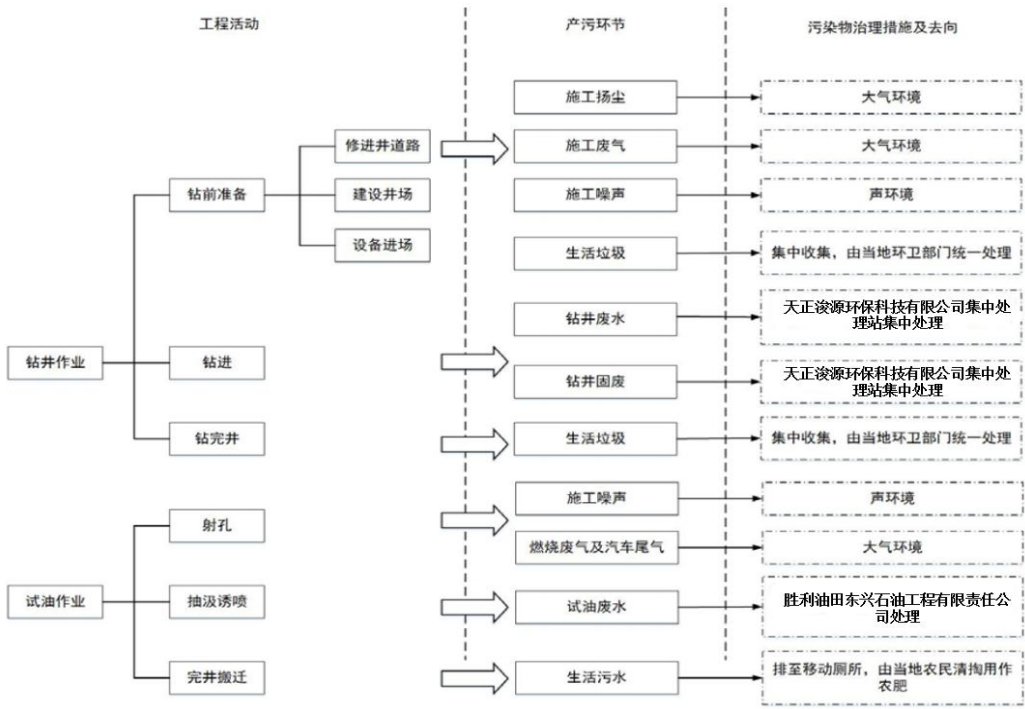
图 3 钻井及试油工艺流程及产污环节图
