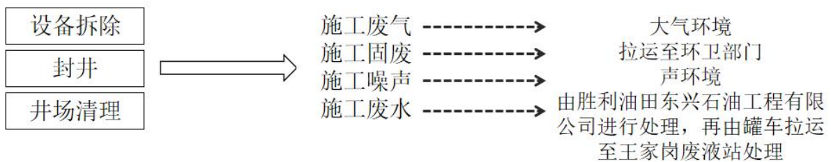
图 4 封井工艺流程及产污环节图
