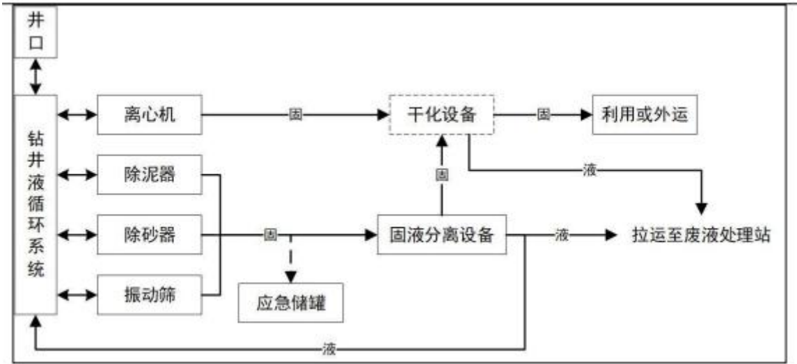
图 5 “泥浆不落地”基本处理工艺流程图
