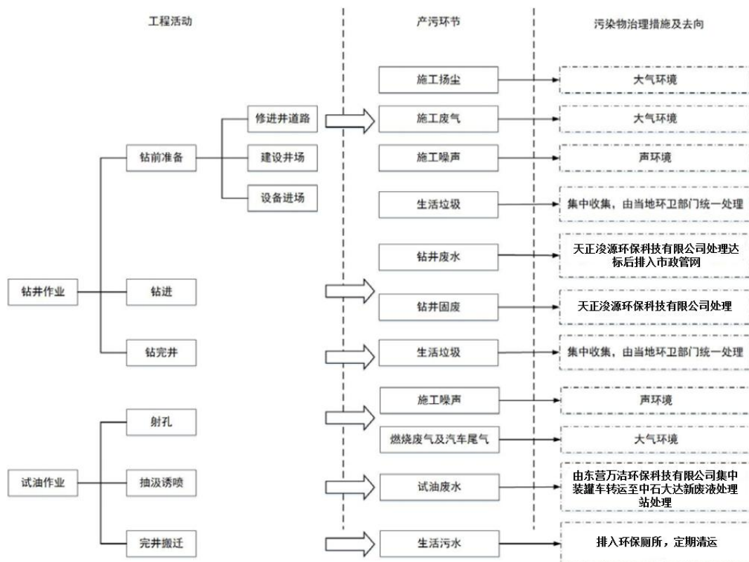
图 3 钻井及试油工艺流程及产污环节图
