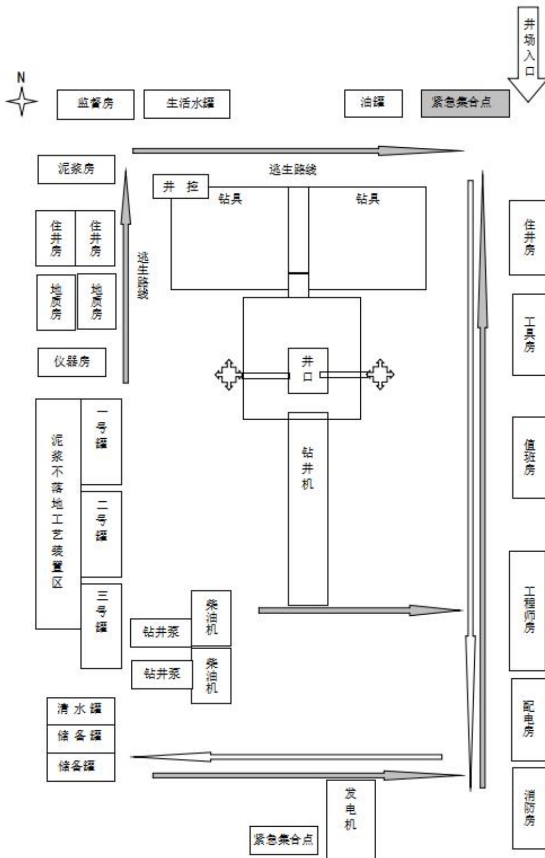
图 2 钻井井场平面布置示意图
