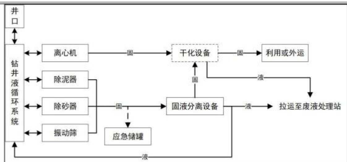
图 5 “泥浆不落地” 工艺原理图
