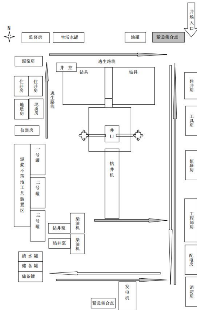
图 2 钻井井场平面布置示意图
