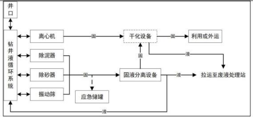
图 5 “泥浆不落地”基本处理工艺流程图
