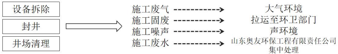
图 4 封井工艺流程及产污环节图
