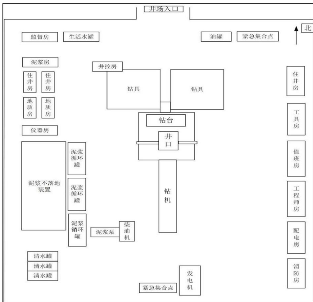
图 2 钻井井场平面布置示意图
