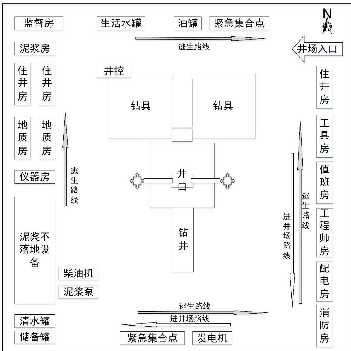
图 2 钻井井场平面布置示意图
