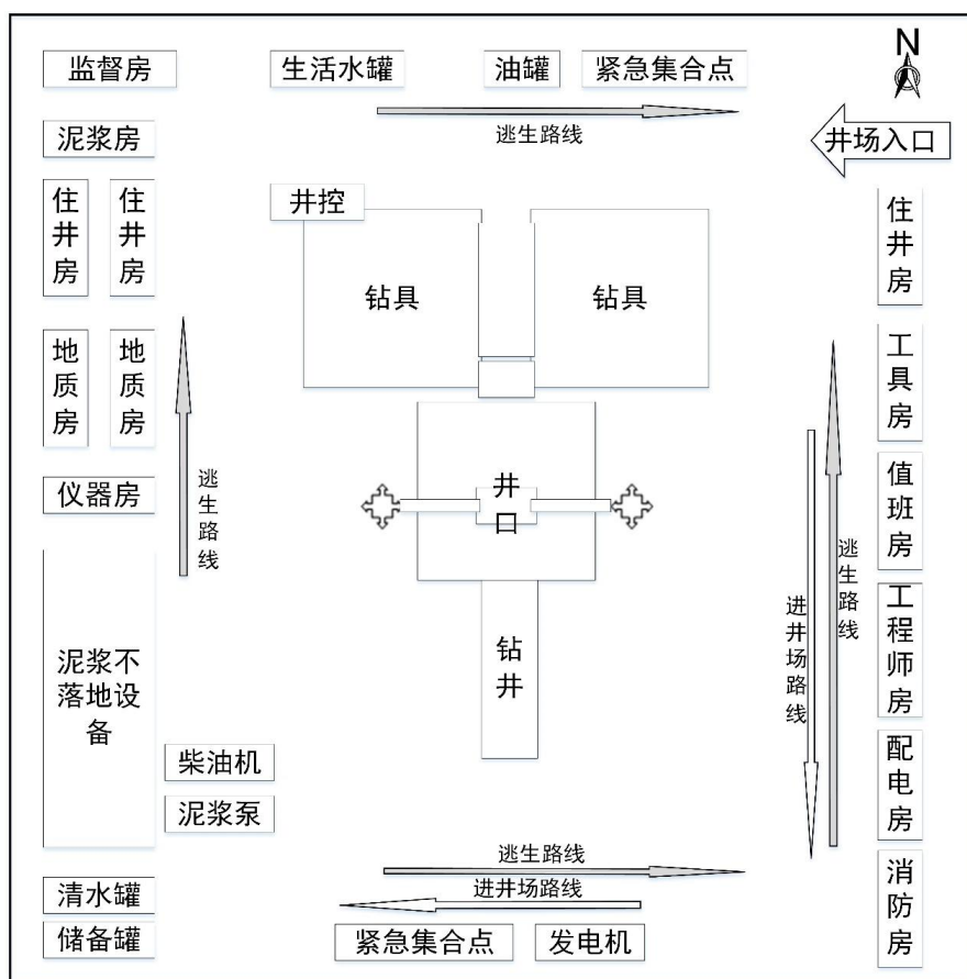
图 2 钻井井场平面布置示意图
