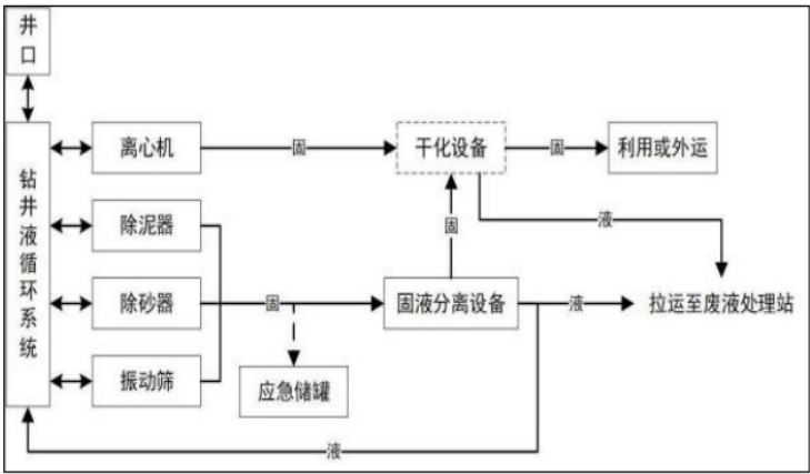
图 2-2 泥浆不落地处理工艺流程示意图
