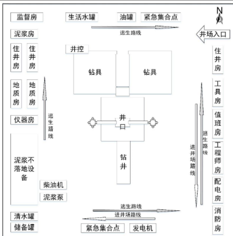
图 2-1 钻井井场平面布置示意图
