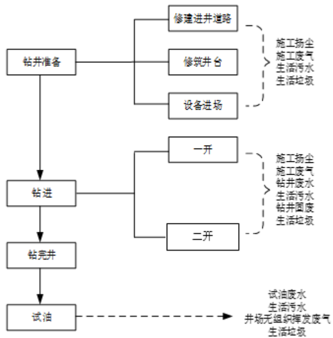
图 2-2 钻井过程和试油工艺流程及产污环节图
