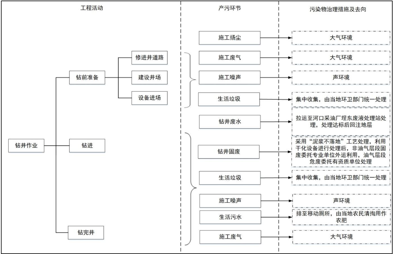
图 2-2 钻井工艺流程及产污环节图
