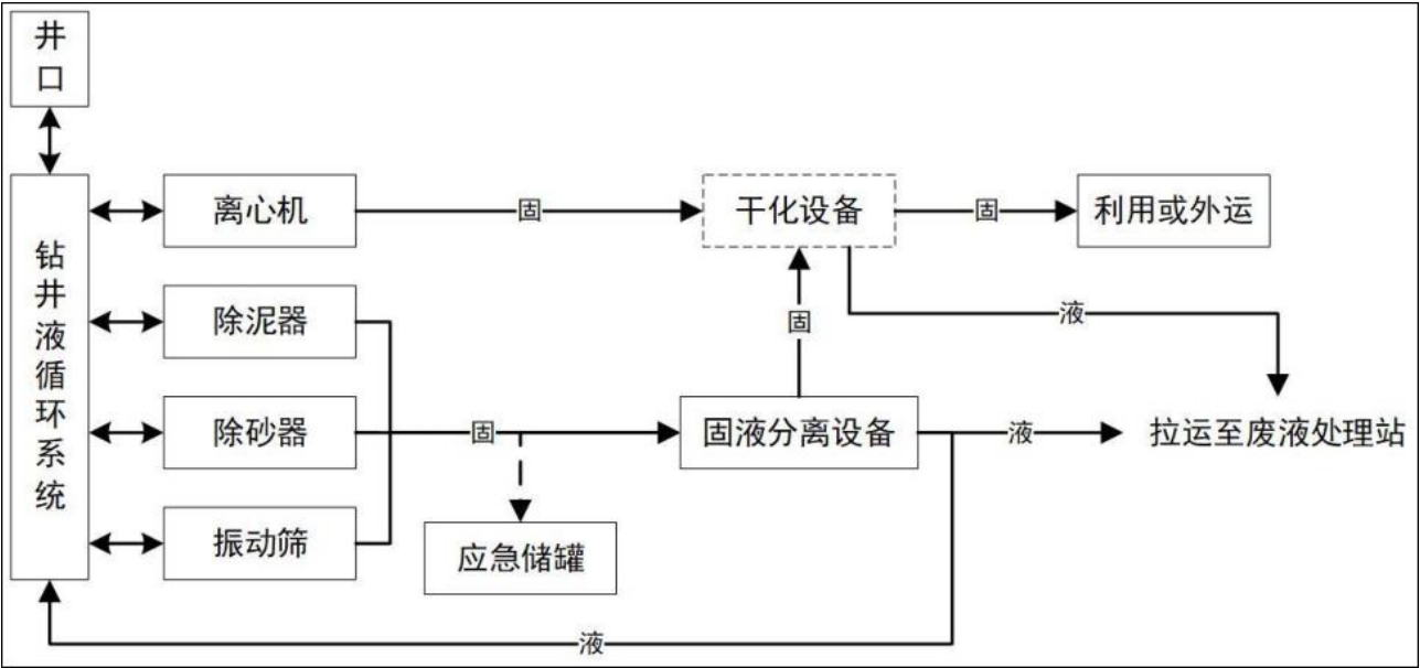
图 2-2 “泥浆不落地”工艺原理示意图
