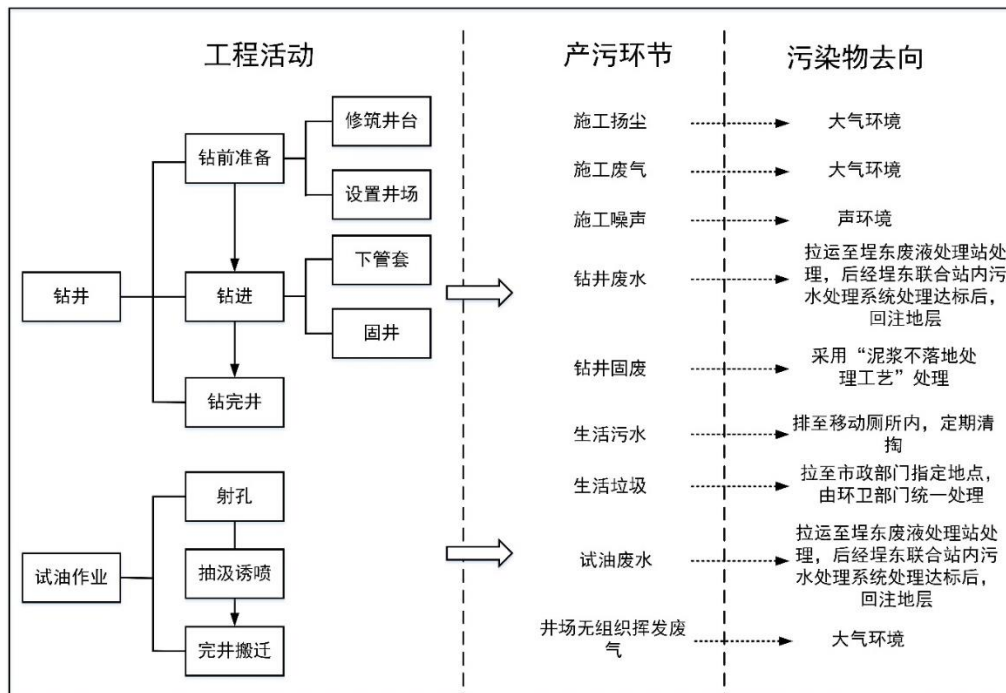
图 3 钻井及试油工艺流程及产污环节图
