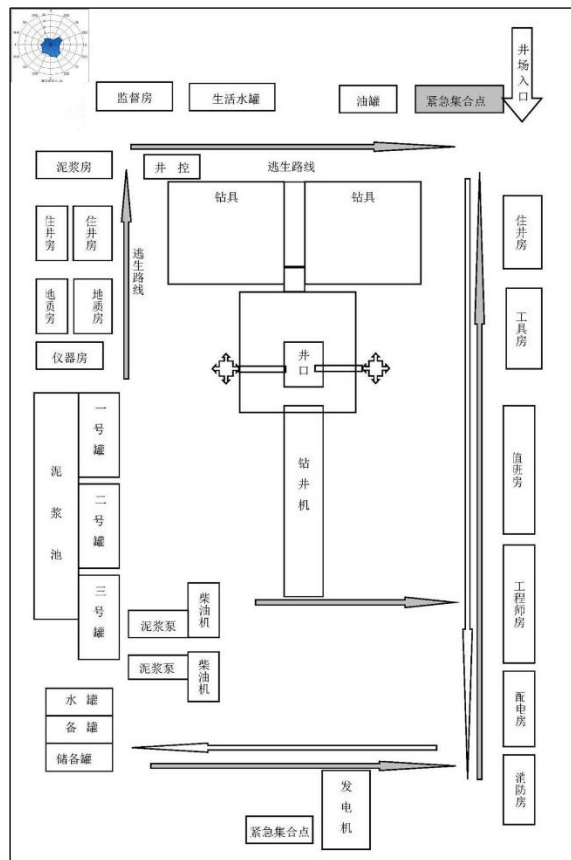
图 2-1 钻井井场平面布置示意图
