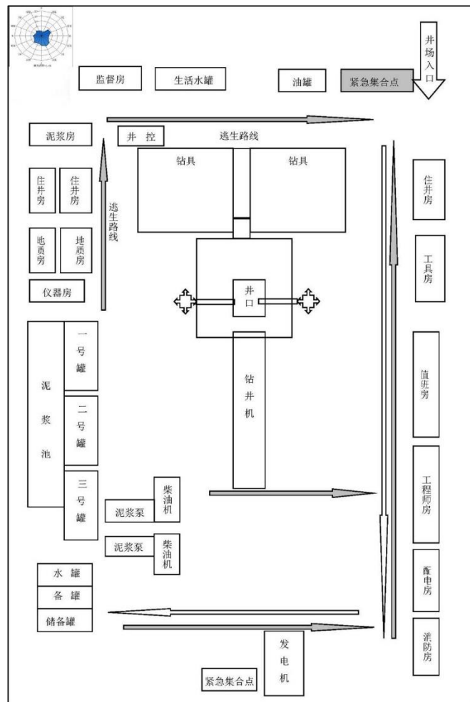
图 2-1 钻井井场平面布置示意图
