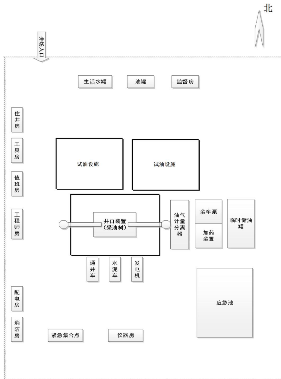
图 2-2 试油过程平面布置图
