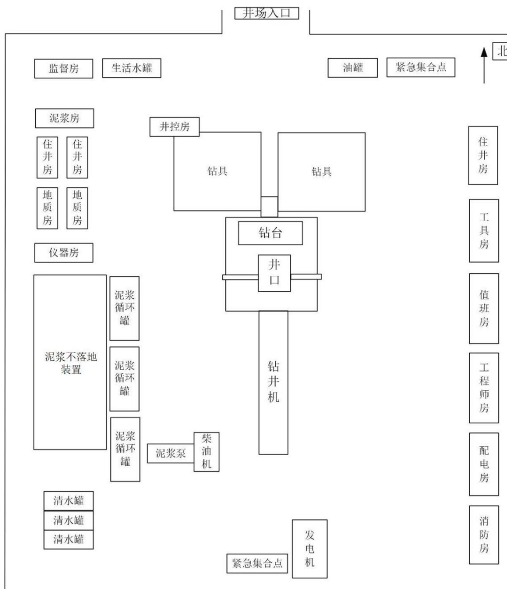
图 2-1 钻井井场平面布置示意图
