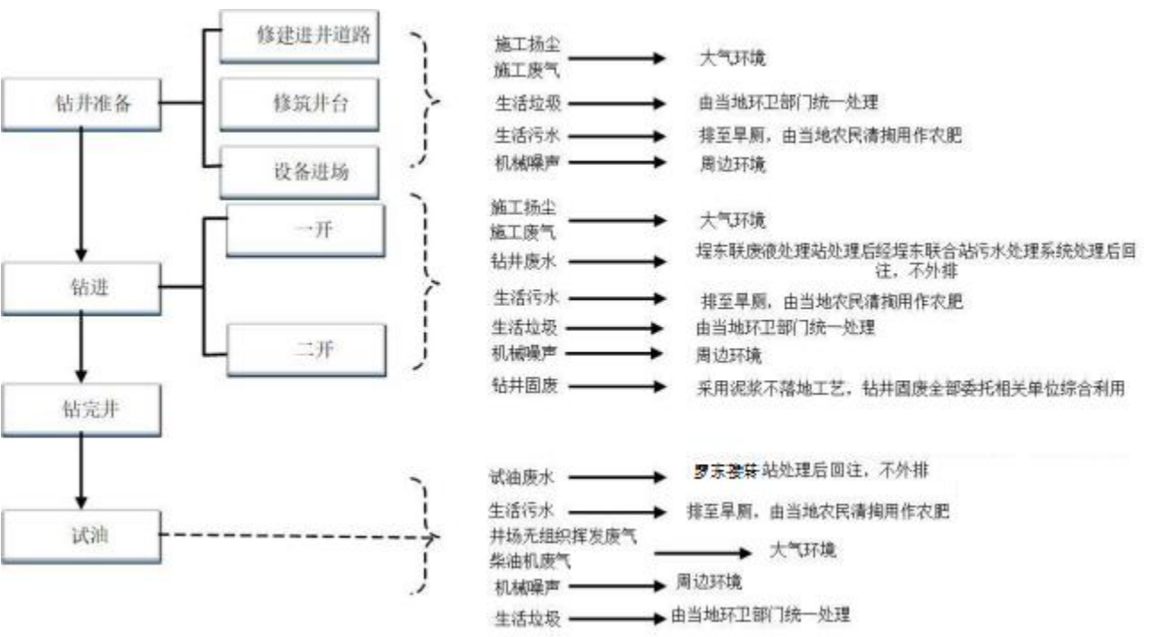
图 3 钻井及试油工艺流程及产污环节图
