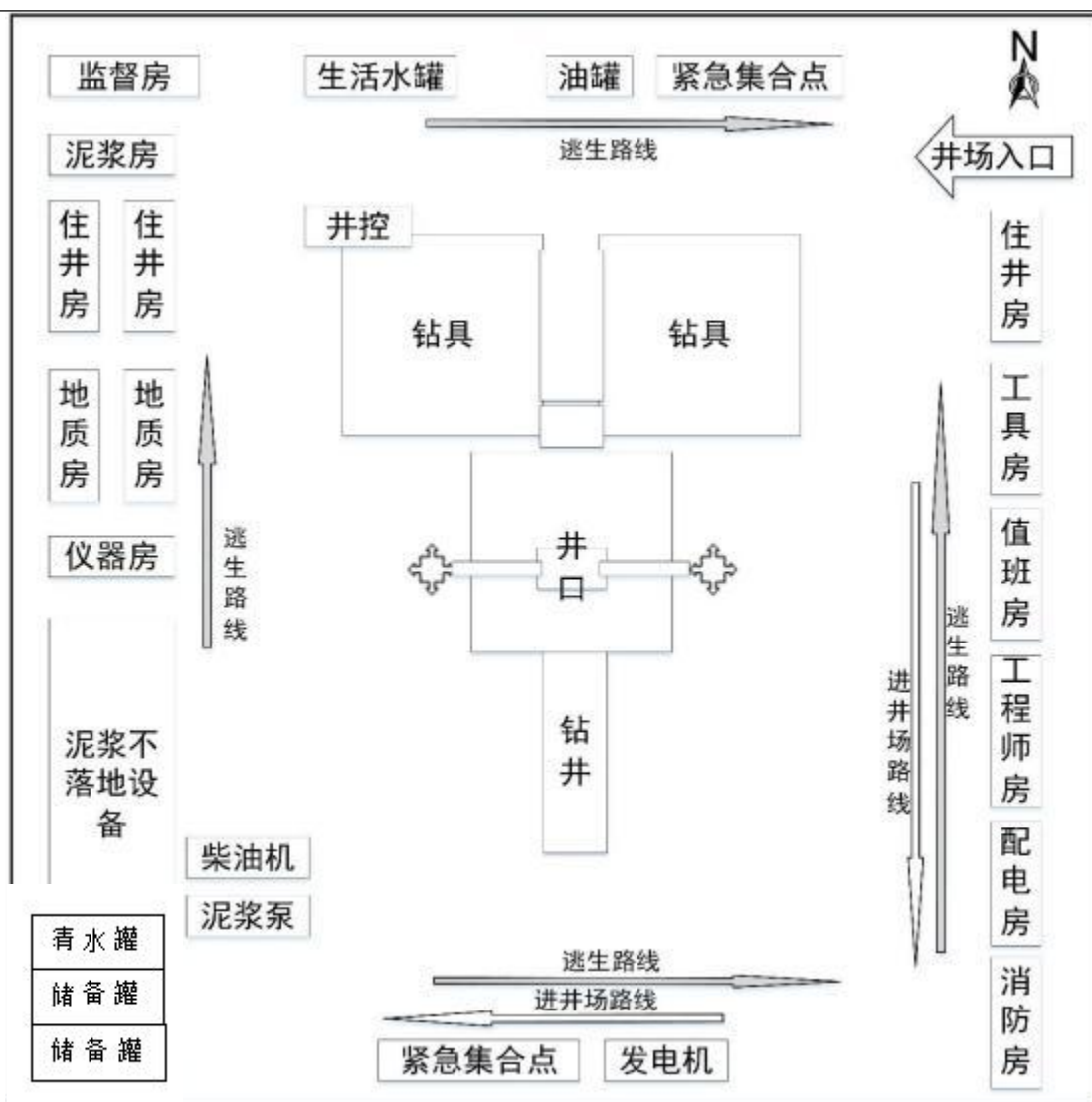
图 1 钻井井场平面布置示意图
