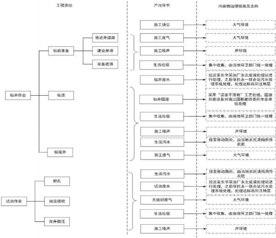
图 4 钻井及试油工艺流程及产污环节图
