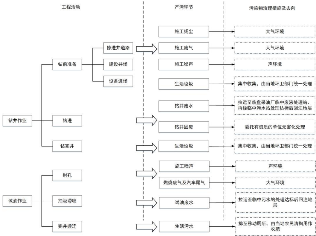
图 2 钻井及试油工艺流程及产污环节图
