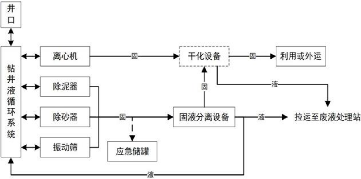
图 4 钻井固体废物处理工艺流程图
