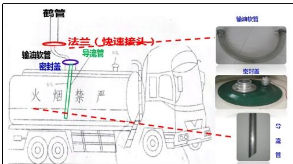
图 3 浸没式装车原理图
