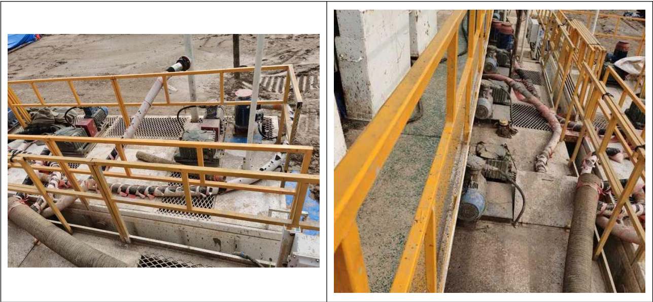
图 5 利 381 井钻井现场泥浆不落地装置照片
