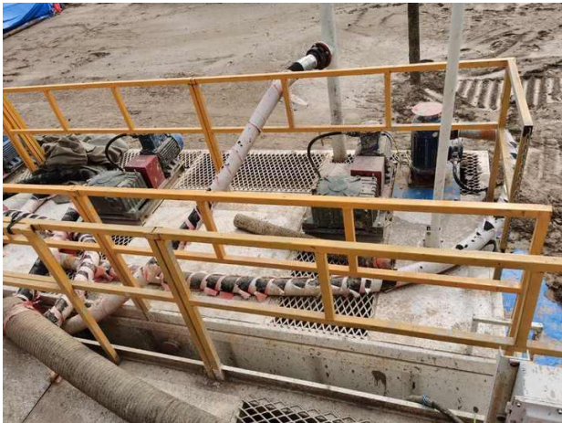
图8 利381井钻井现场泥浆不落地装置照片
