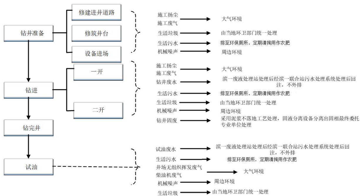
图 2 钻井及试油工艺流程及产污环节图
