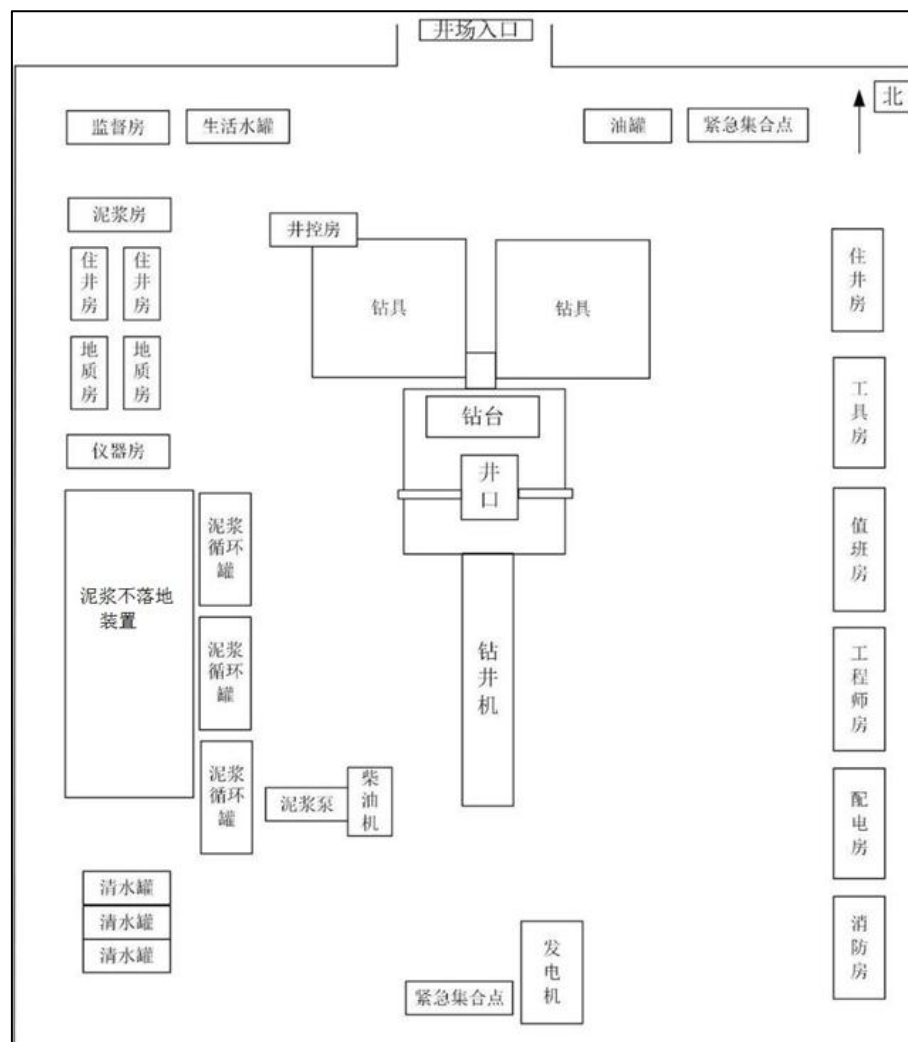
图 1 钻井井场平面布置示意图
