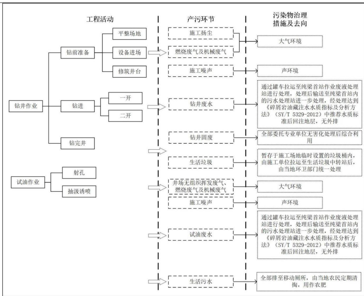
图2 钻井及试油工艺流程及产污环节图
