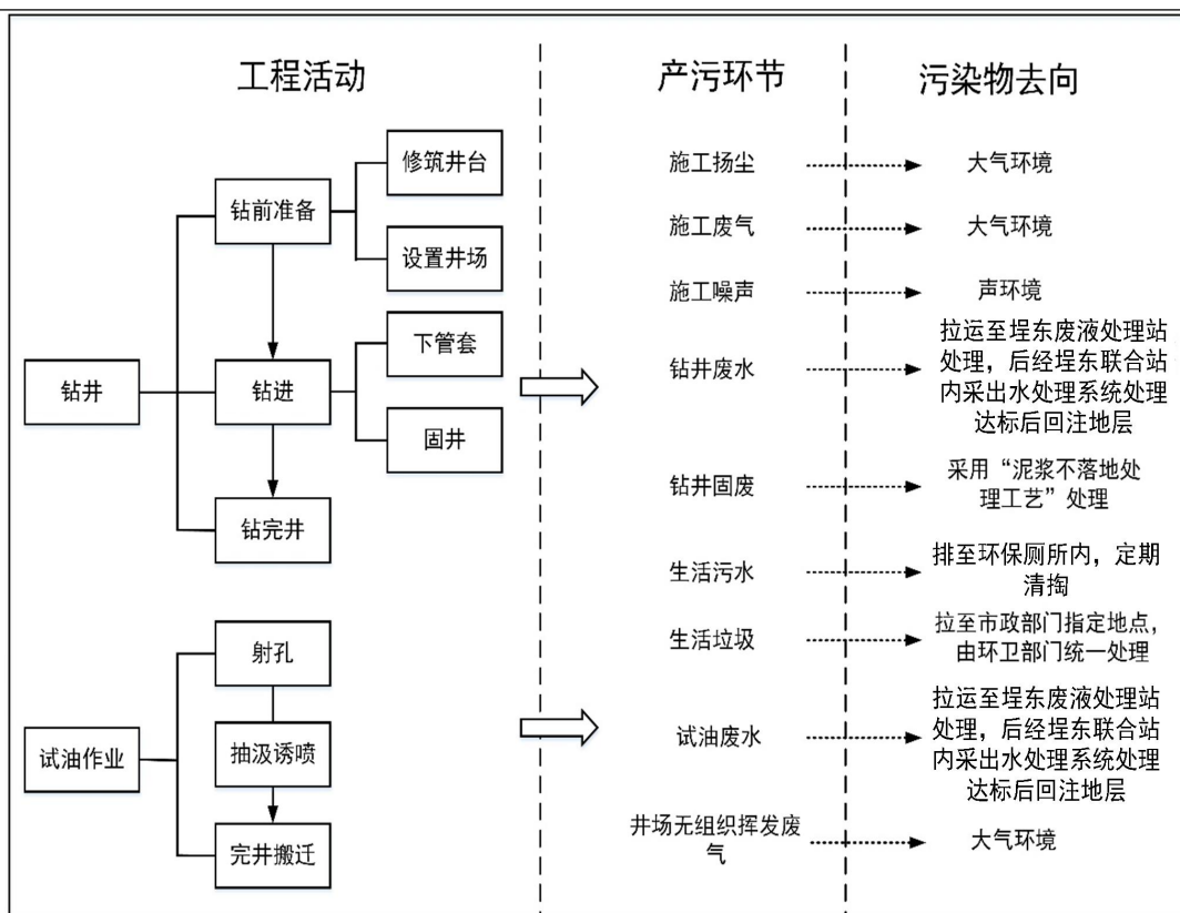
图2 钻井及试油工艺流程及产污环节图
