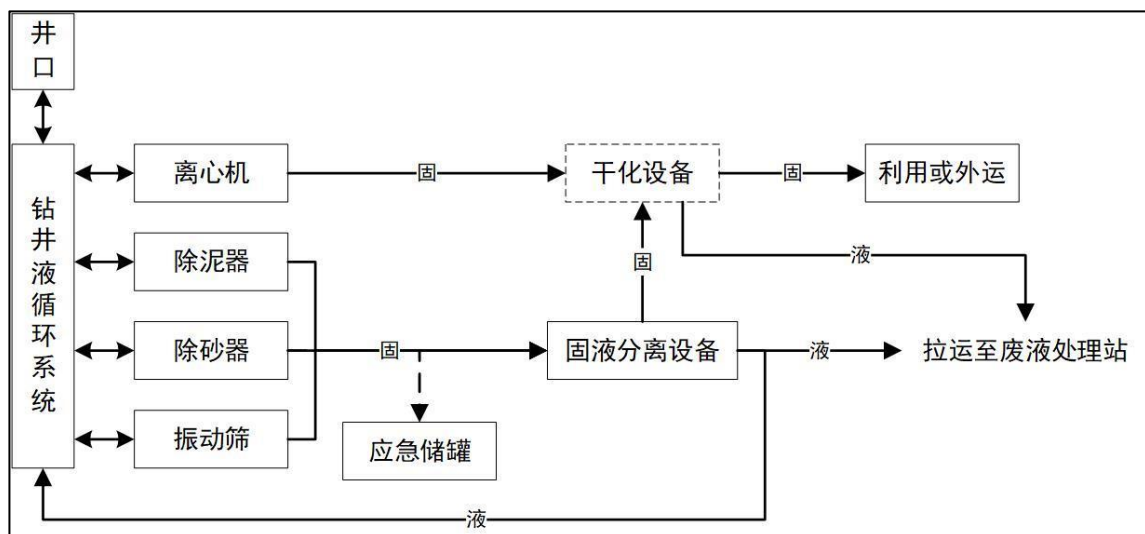
图 6 “泥浆不落地”工艺原理示意图
