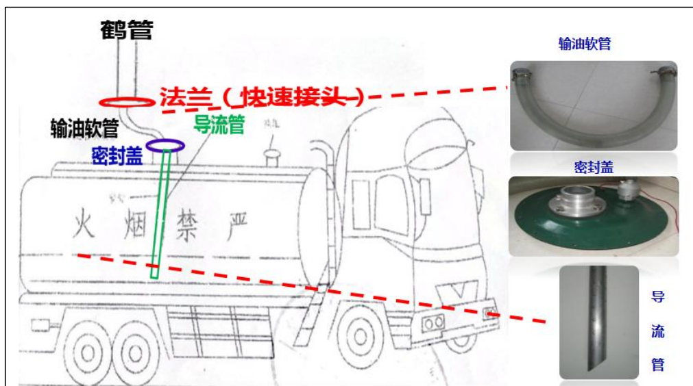
图 5 浸没式装车原理图
