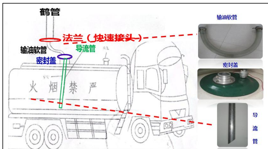
图2-4 浸没式装车原理图
