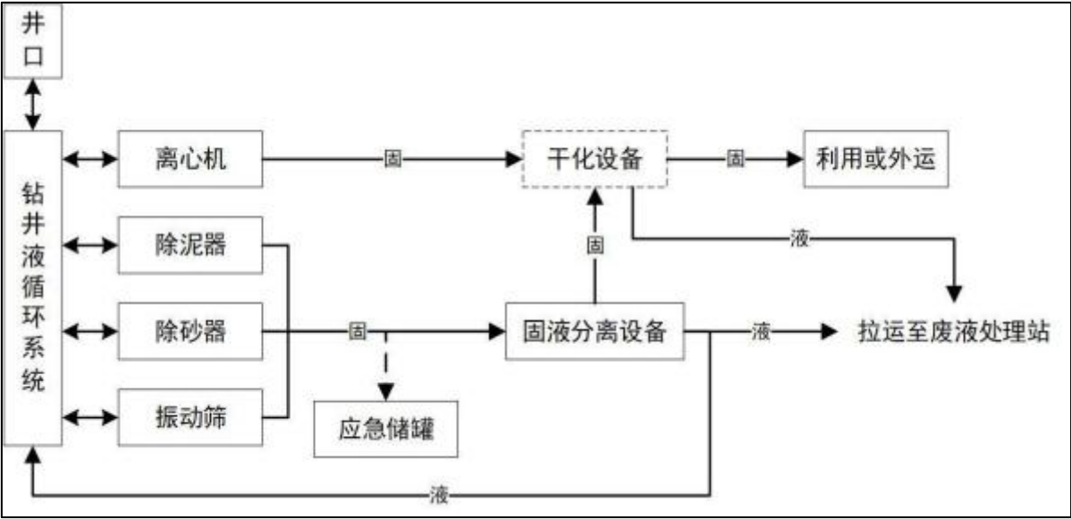
图2-5 “泥浆不落地”工艺流程示意图
