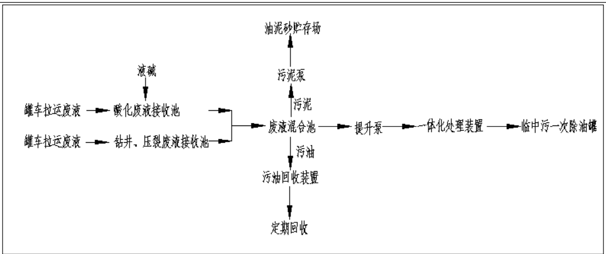
图 5-2 临盘采油厂废液处理站工艺流程
