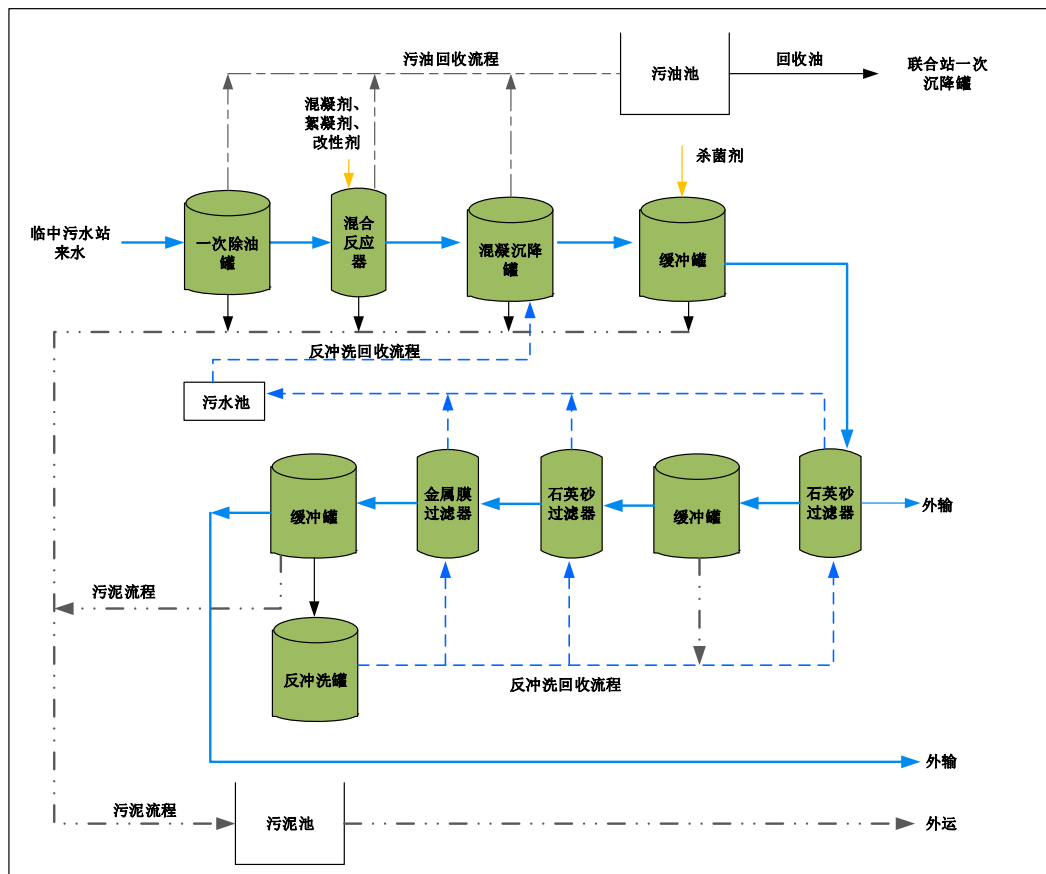
图 5-2 临盘采油厂废液处理站工艺流程
