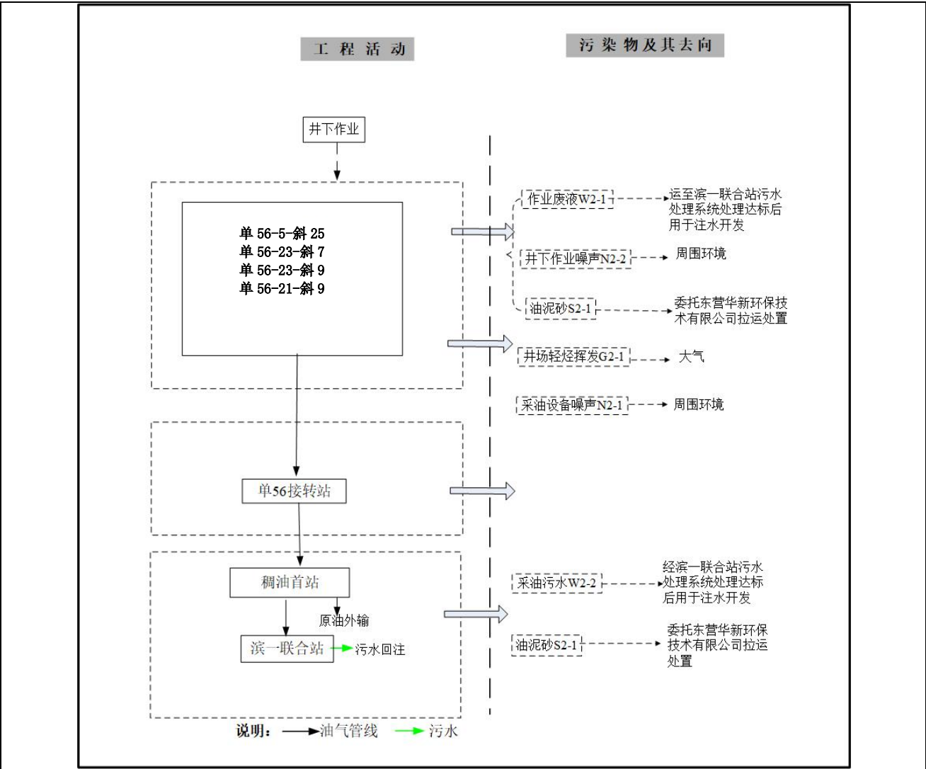
图 3-4 运营期工艺流程及产污环节图
