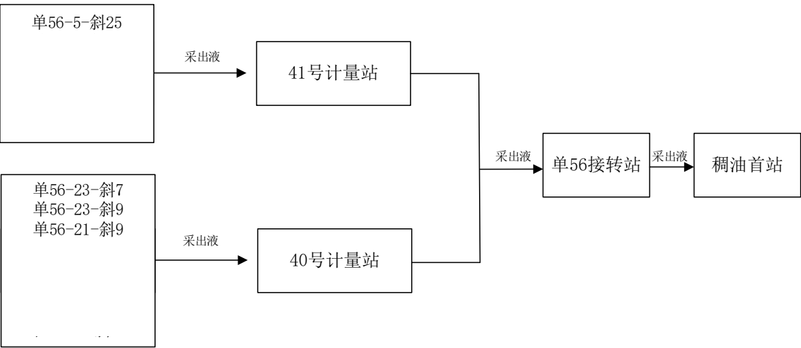
图 3-2 集输流程
