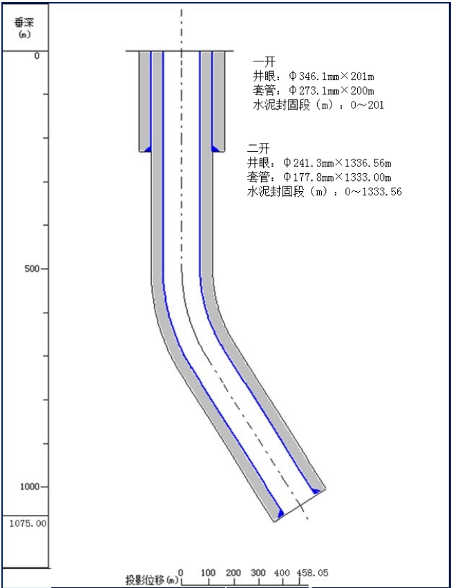
图 3-1 井身结构示意图
